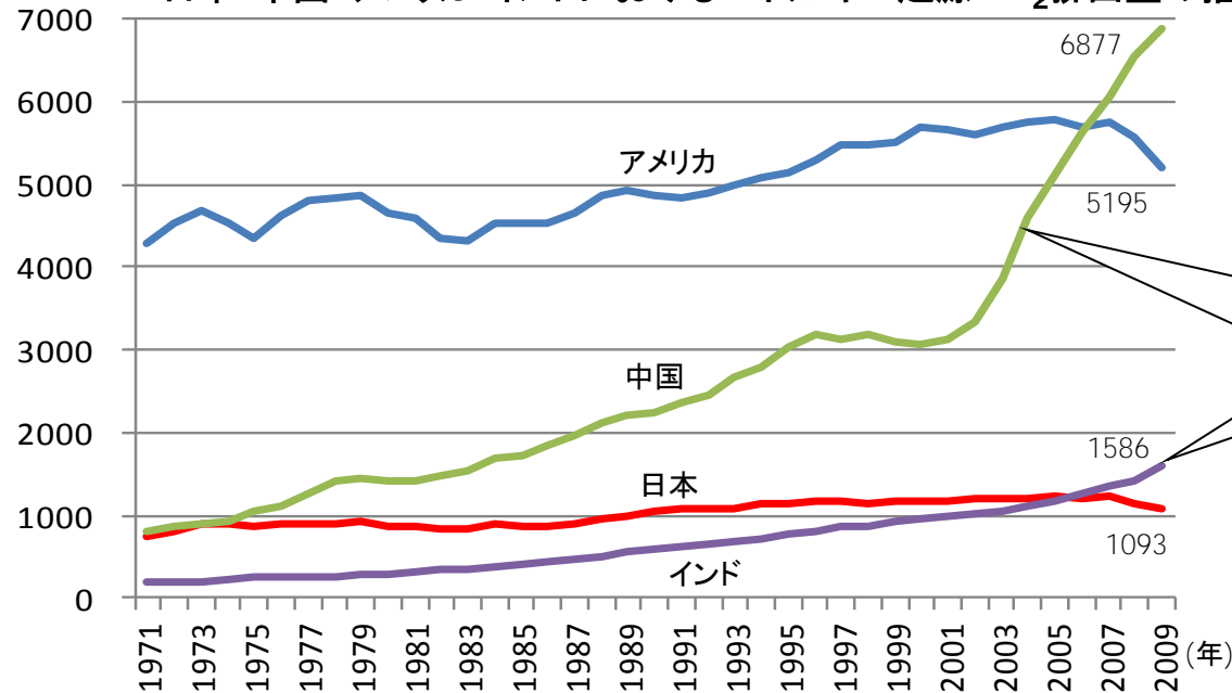
(Mt-CO 2 ) 日本・中国・アメリカ・インドにおけるエネルギー起源CO 2 排出量の推移
