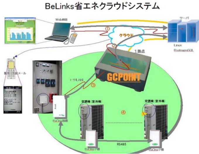
図 3-2 サイクリック制御の遠隔操作システム
