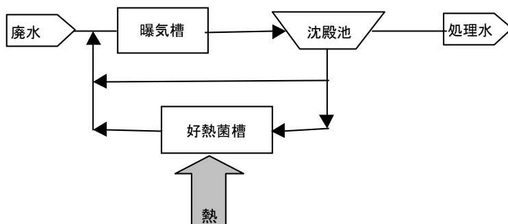
図 2-7-9 好熱菌による汚泥減容化プロセス
