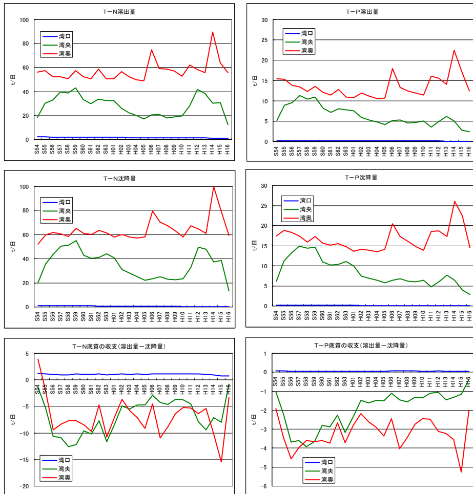
図 49 東京湾における窒素、りん溶出量・沈降量とその差の推移(計算値)
