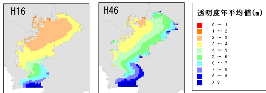
図 46 東京湾における各水質項目の分布図(計算値)
