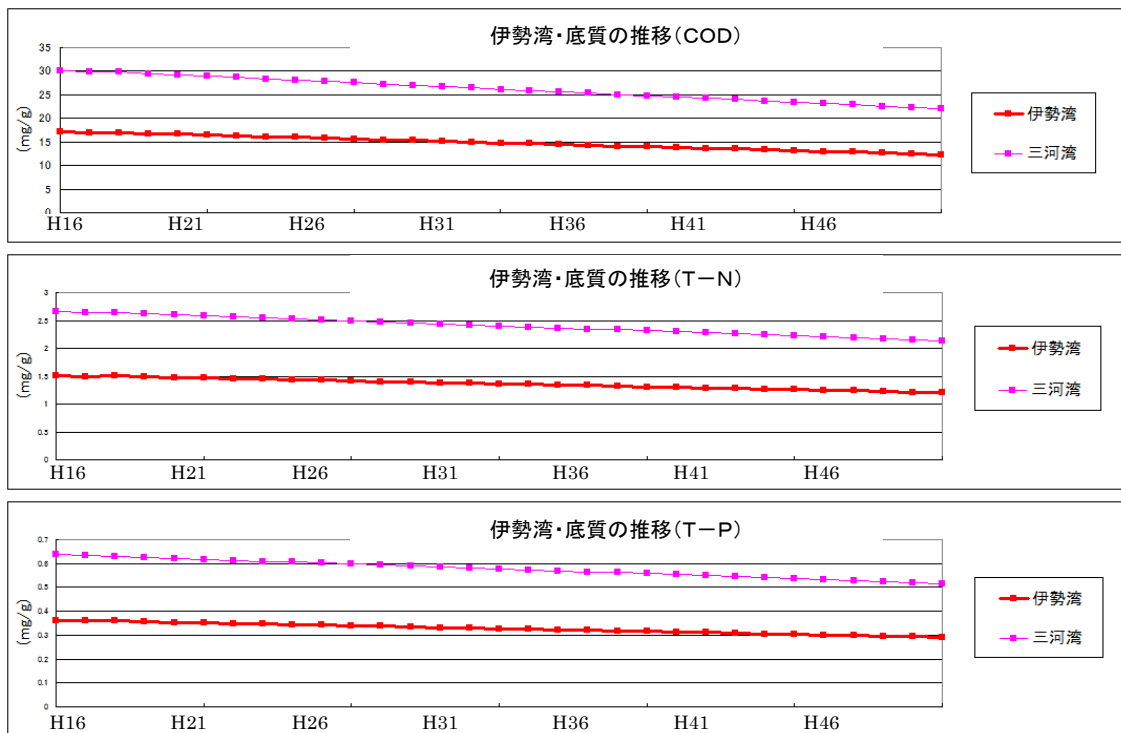
図51 底質(計算値)の推移(伊勢湾)
