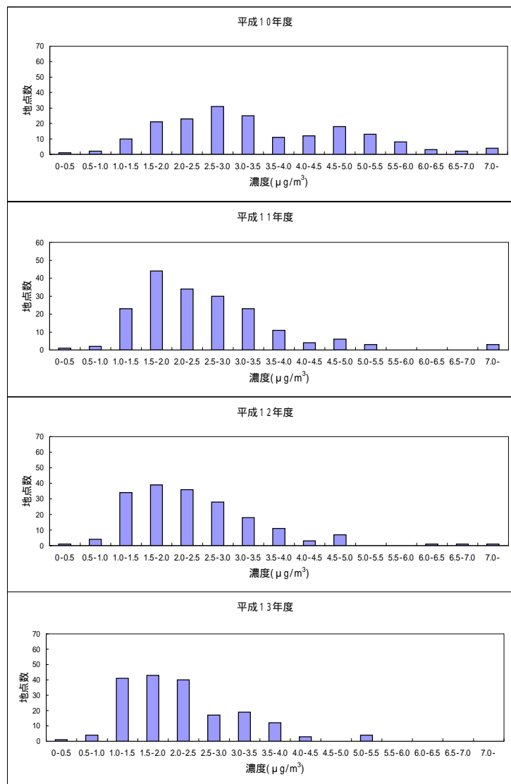
継続測定地点におけるベンゼンの大気環境中濃度分布の推移
