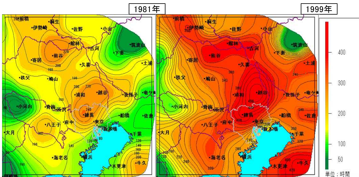
図3 東京地域における30°C超延べ時間の広がり(出典:環境省) 1981年と1999年の7月から9月の各地点のアメダスデータから30°Cを超えた延べ時間数を集計し、分布を等時間線で示したもの。
