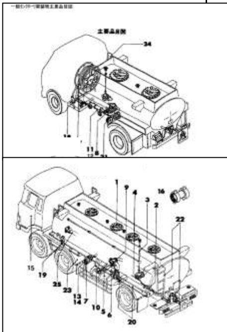
一般タンクローリ架装物解体マニュアル タンク本体、配管材質：鉄、アルミ、ステンレス
