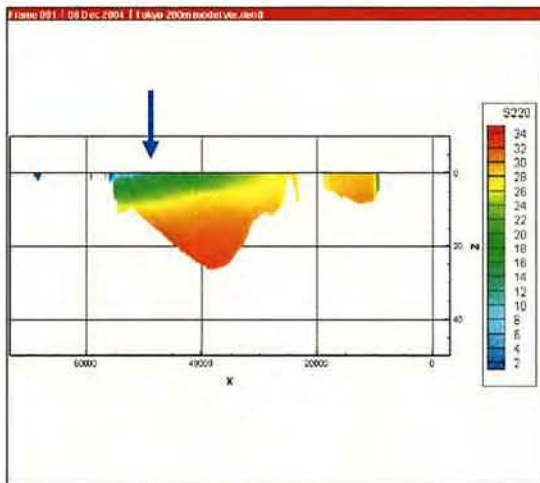
南北断面
