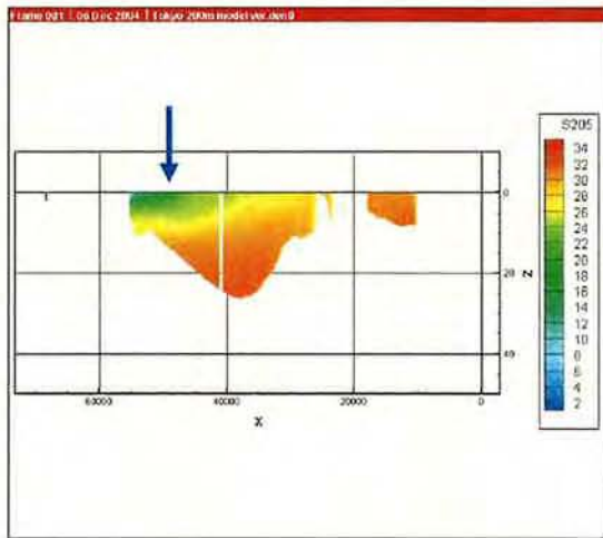
南北断面
