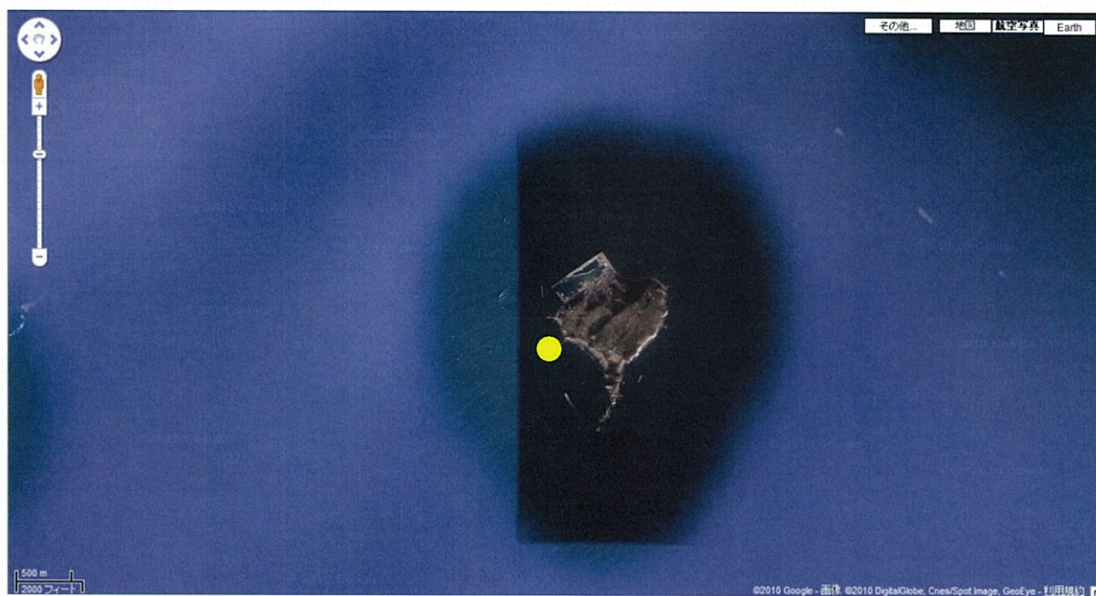
図 6. 13 (4) 沿岸域 (伊勢湾 St. 4 湾口 3)
