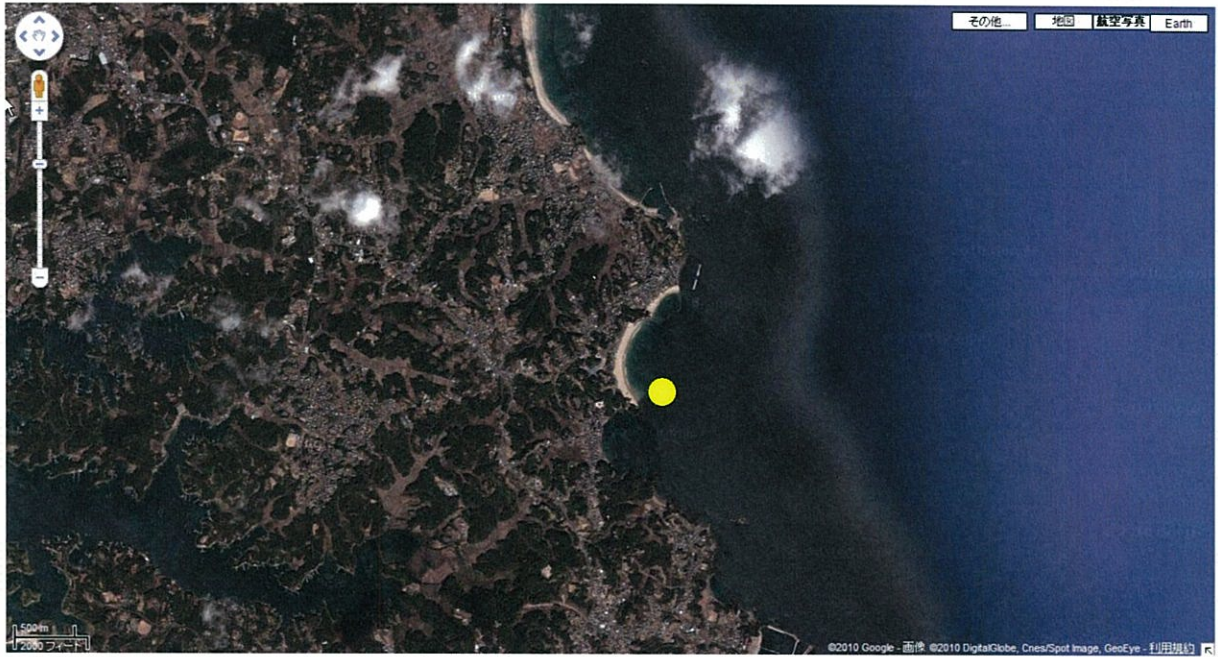
図 6. 13 (1) 沿岸域 (伊勢湾 St.1 湾口 1)
