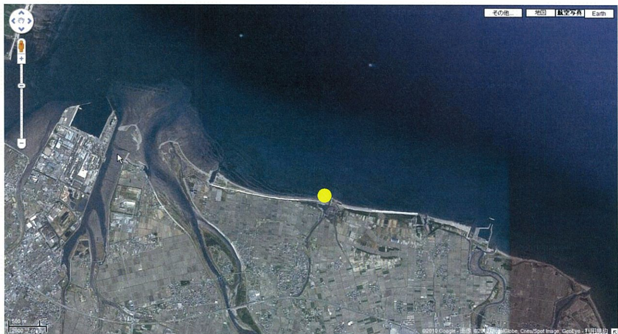
図 6. 13 (6) 沿岸域 (伊勢湾 St. 8 松坂藻場)
