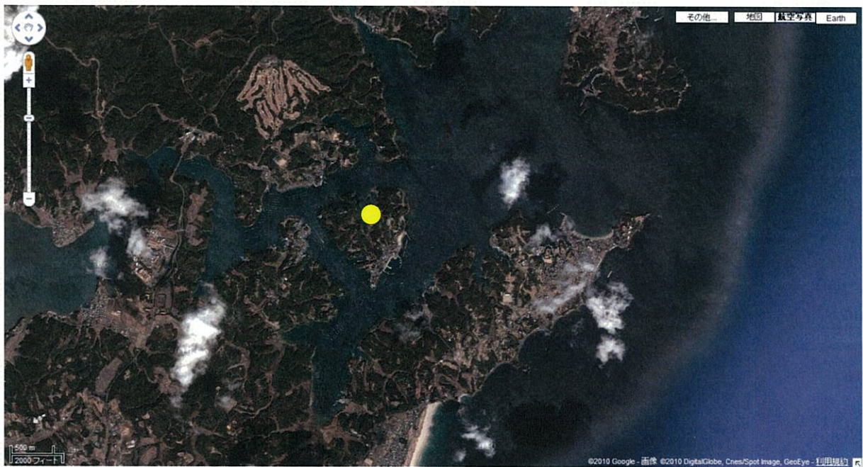
図 6. 13 (2) 沿岸域 (伊勢湾 St.2 的矢湾)
