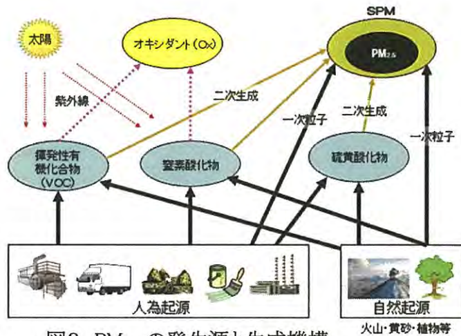
図3 PM 2.5 の発生源と生成機構
