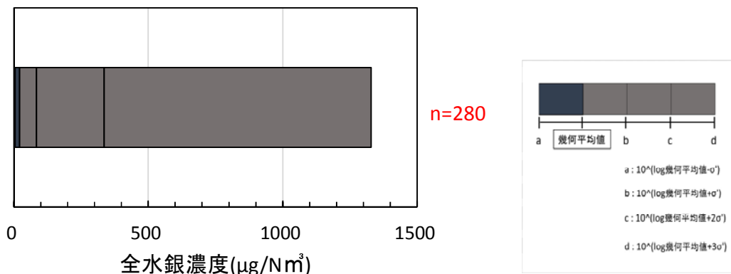
図 II-5-12 セメントクリンカー製造設備の排ガス中全水銀濃度（対数標準偏差） （環境省法以外）
