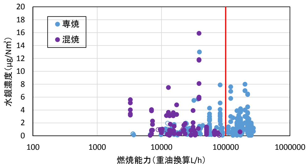
図Ⅱ-1-8 燃烧能力と全水銀濃度 (環境省法のデータ及び環境省法以外のデータを全てプロット)
