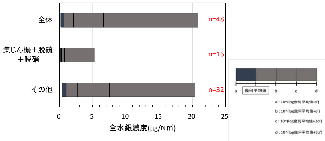
図 II-1-22 排ガス処理設備の種類ごとの水銀濃度（対数標準偏差） （小型石炭混焼ボイラー）（環境省法以外）
