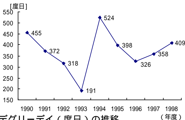
図 20 冷房デGREEデー (度日) の推移
