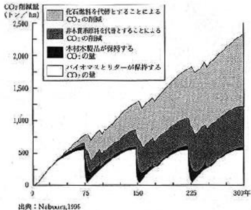
図 28 ヨーロッパでのノルウェイトウヒの造林によって達成されるCO 2 の吸収と排出量の削減(累積t CO 2 /ha)
