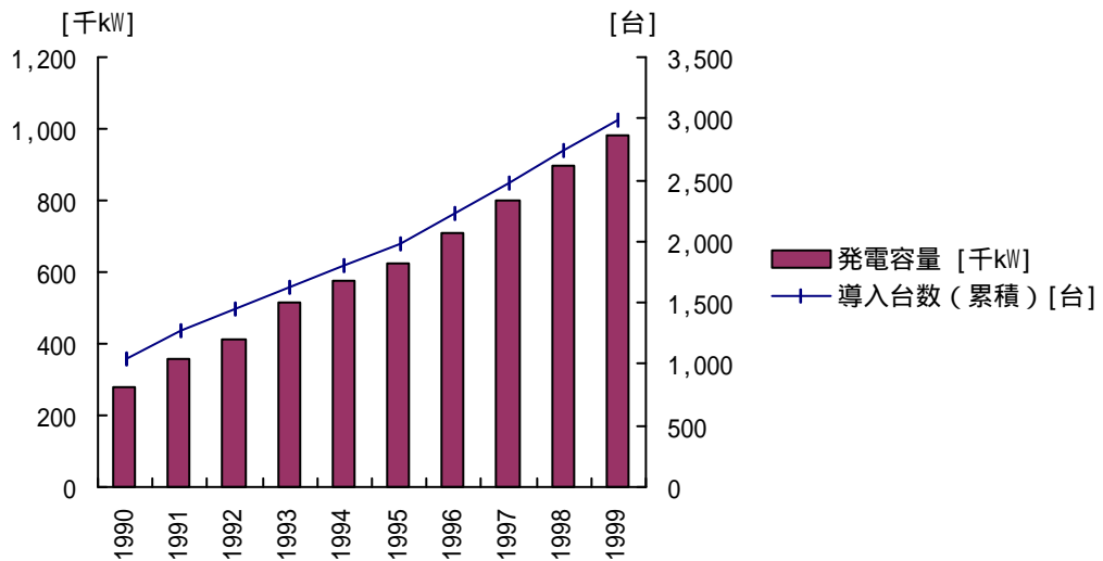
図 71 民生用コージェネレーションの普及状況
