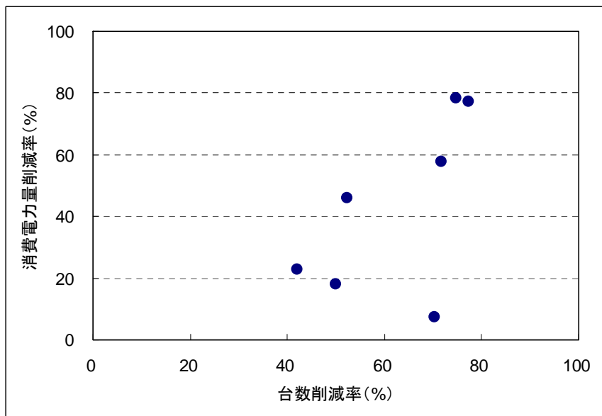
図2 機器台数削減率と消費電力量削減率の関係
