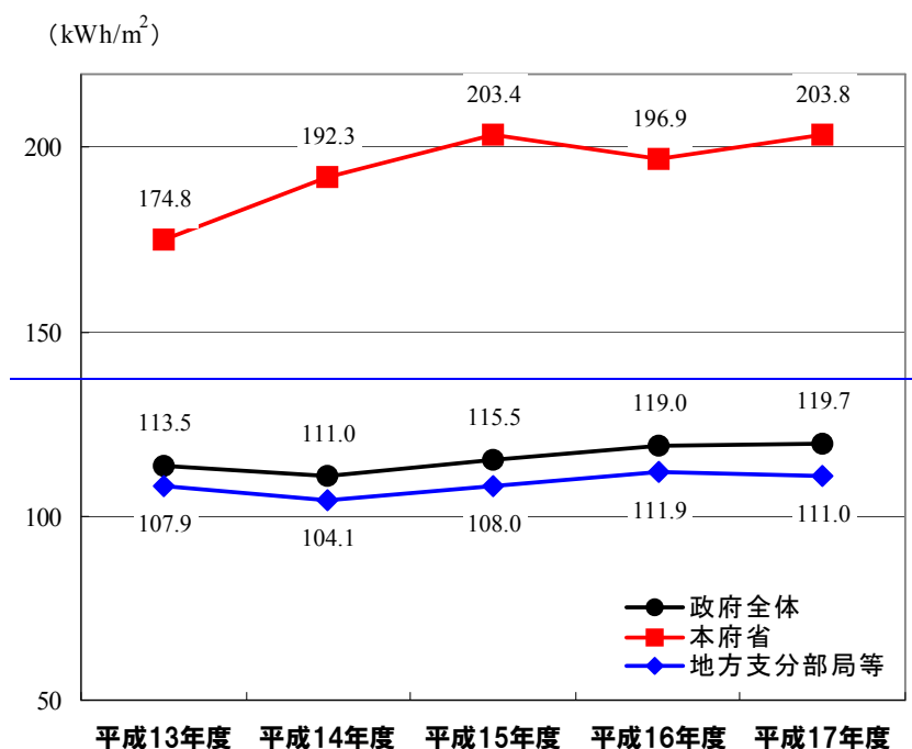
図VI-1-2 事務所の単位面積当たり電気使用量の推移
