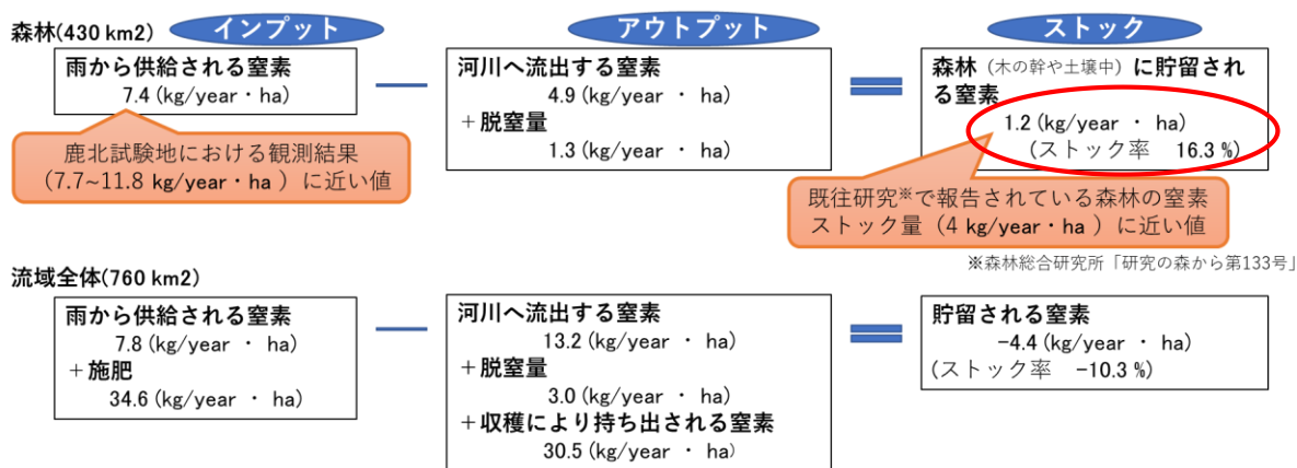
図 12 窒素のインプットに対するストック機能の算定結果
