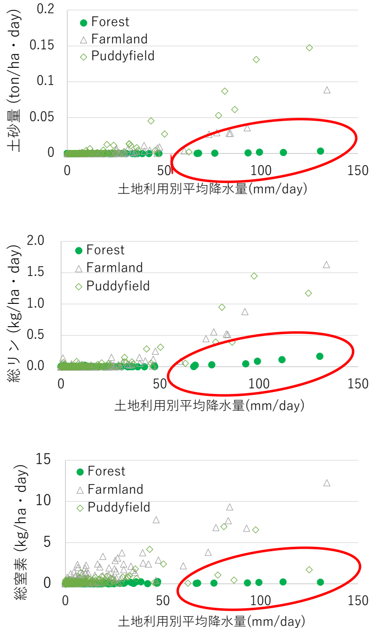
図 9 出水時の土地利用別平均降水量と土砂量、リン、窒素の流出量との関係
