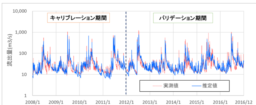
図 3 水流出量の実測値と推定値の推移
