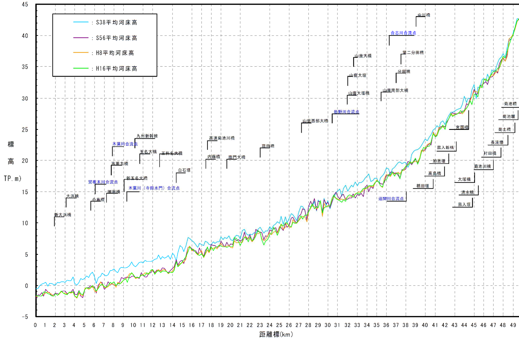
図 18 菊池川の平均河床高縦断面図 6)
