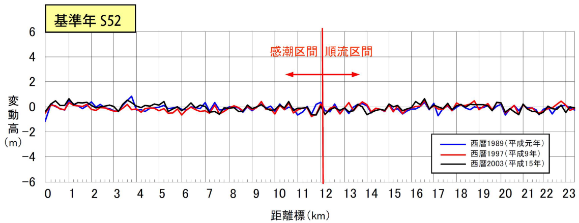
図 16 牛津川の平均河床高の推移 4)
