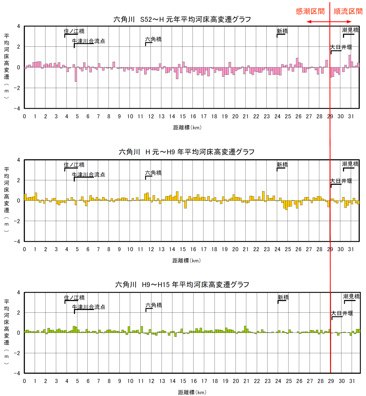
図 15 六角川の平均河床高の変遷(年代別) 4)
