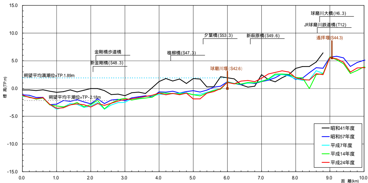
図 22 球磨川下流の平均河床高縦断図
