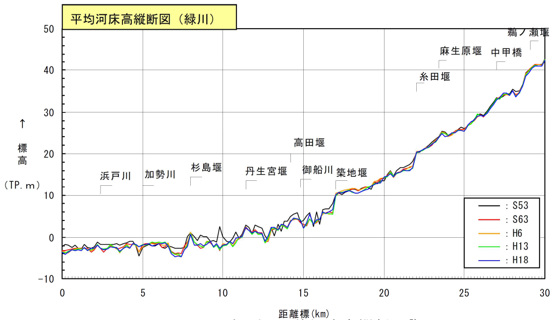
図 20 緑川の平均河床高縦断図 5)
