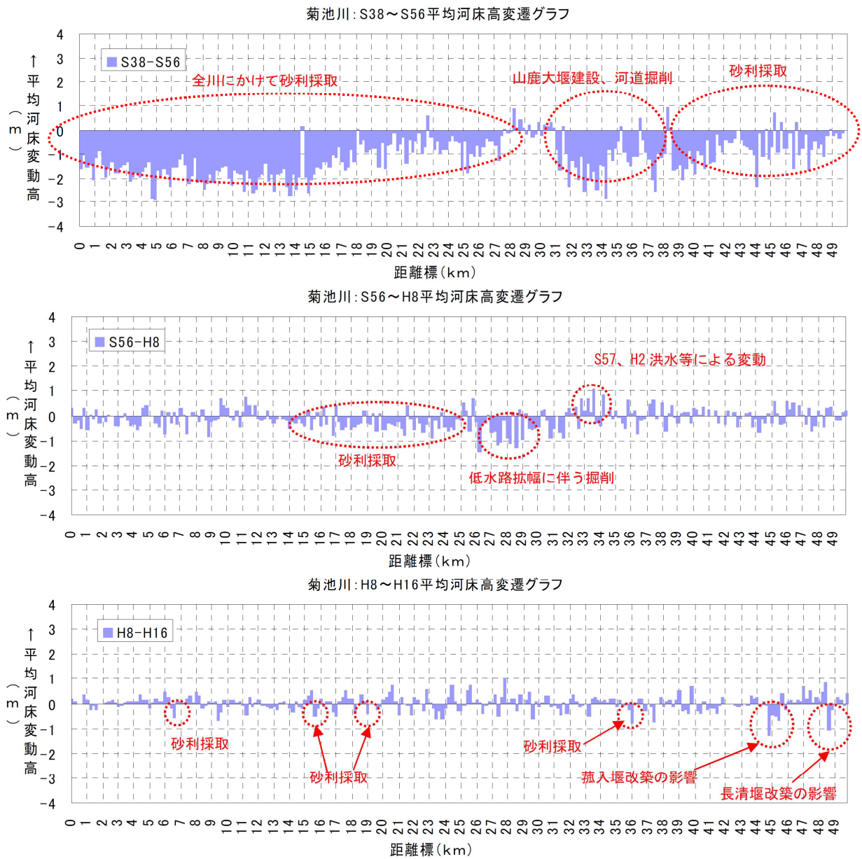
図 19 菊池川の河床変動傾向 6)
