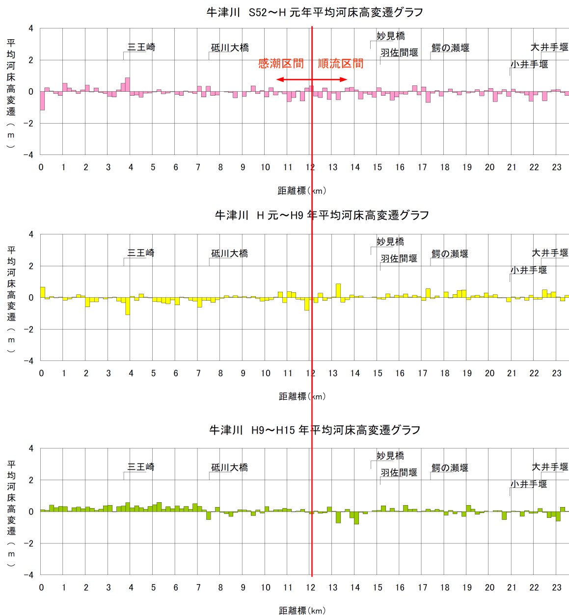
図 17 牛津川の平均河床高の変遷(年代別) 4)
