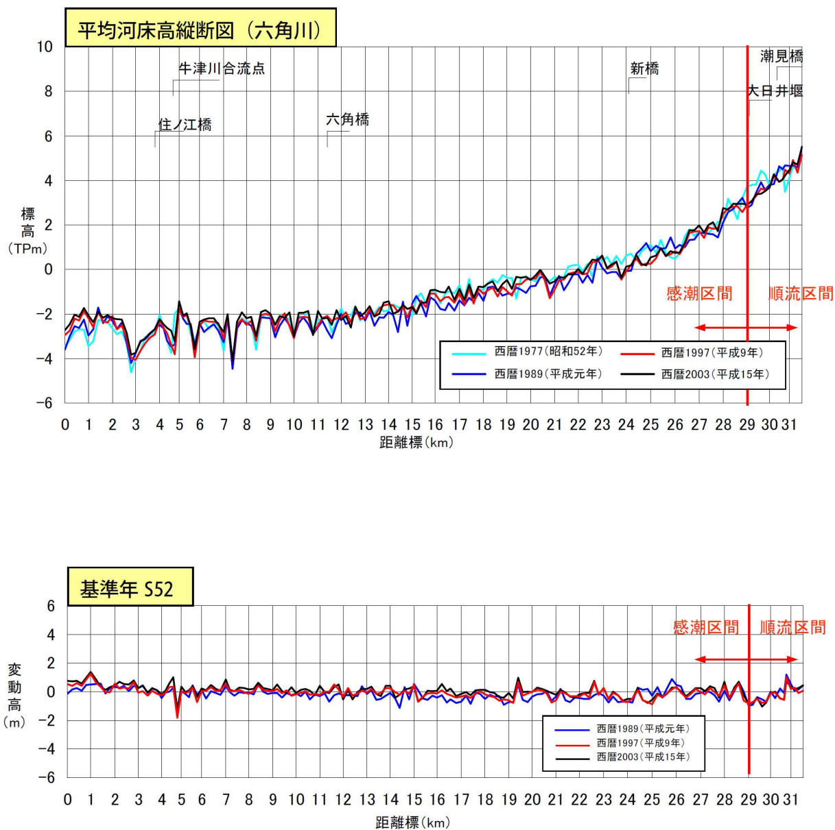
図 14 六角川の平均河床高の推移 4)
