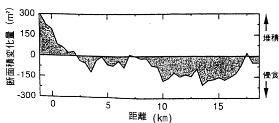
図-8 筑後川感潮域における出水前後の断面積変化
