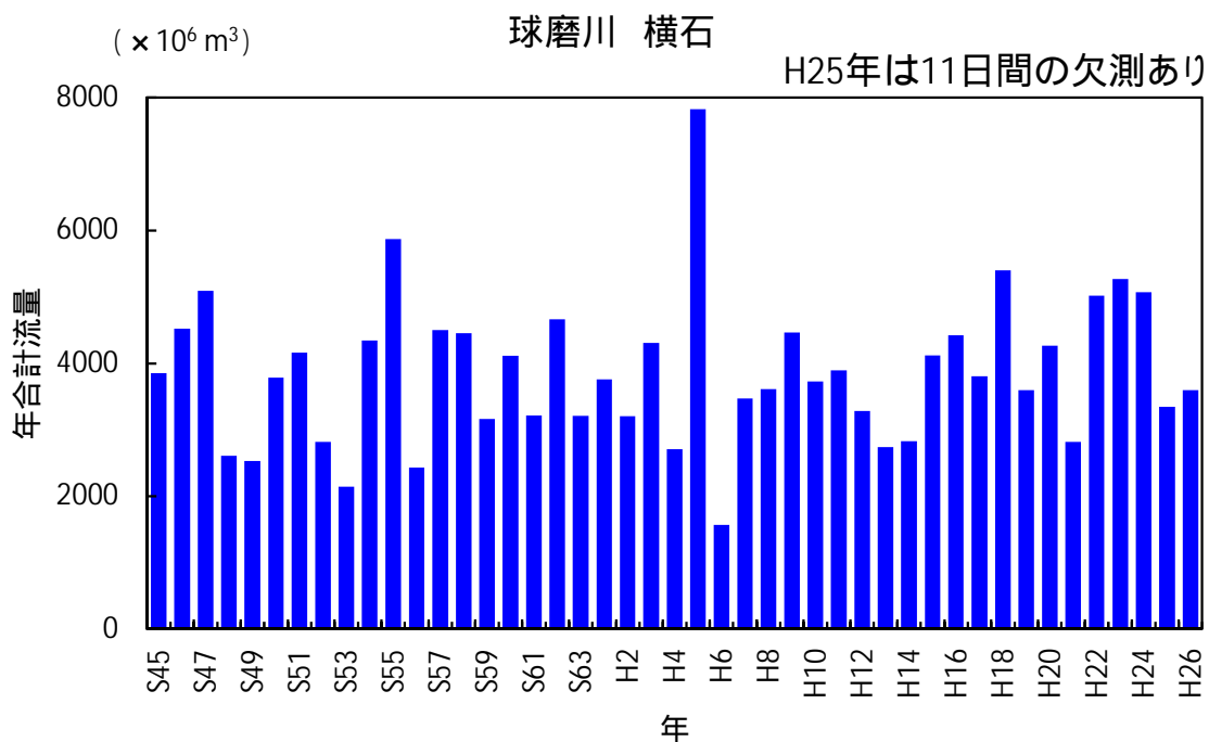
図4 球磨川の年間総流量の推移 1)
