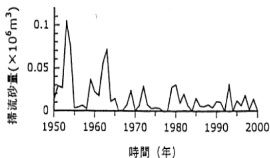
図6 掃流砂量（芦田・道上式による推計値）の経年変化（25.5km 地点）
