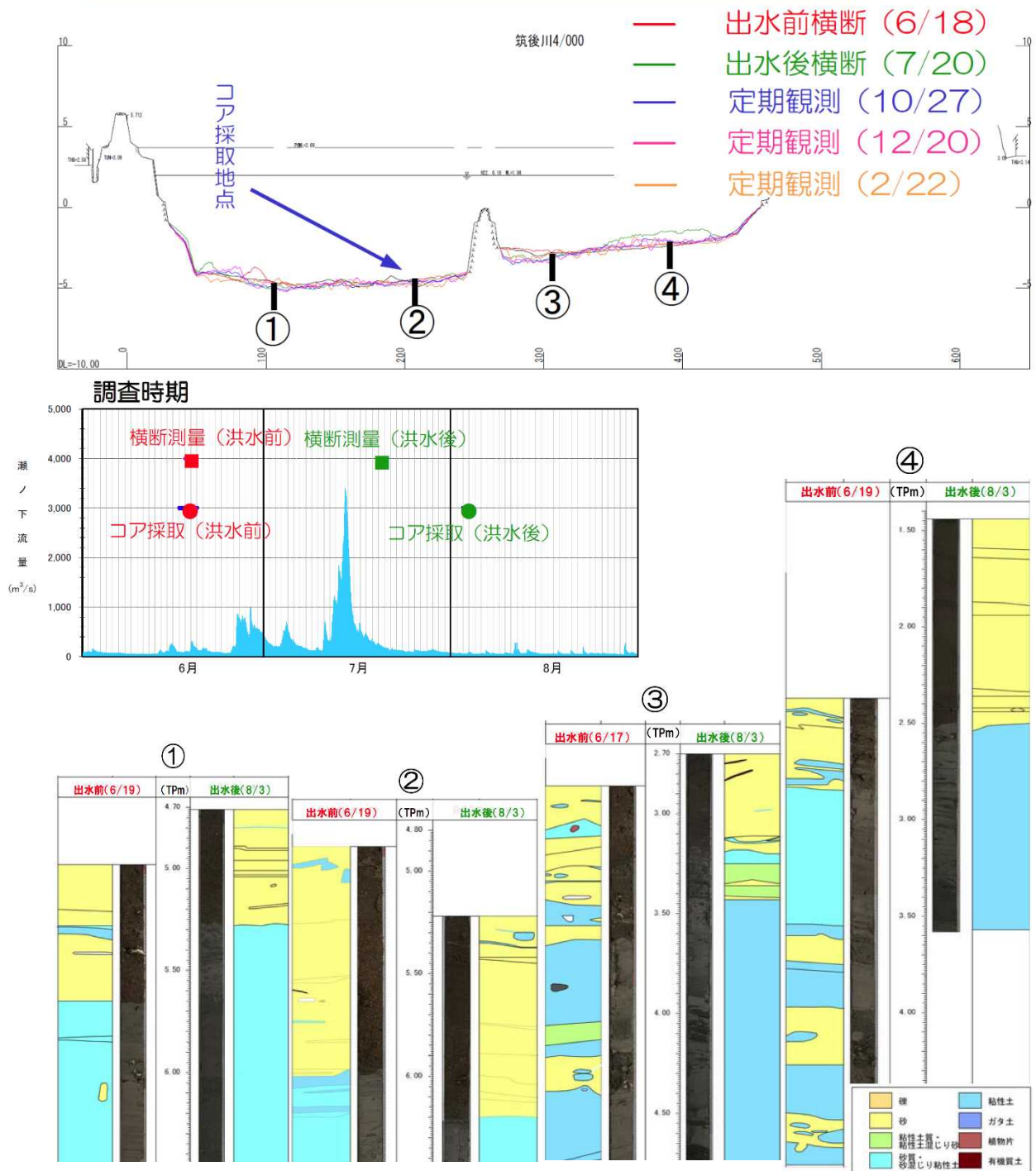
図5 筑後川の河床材料の変化
