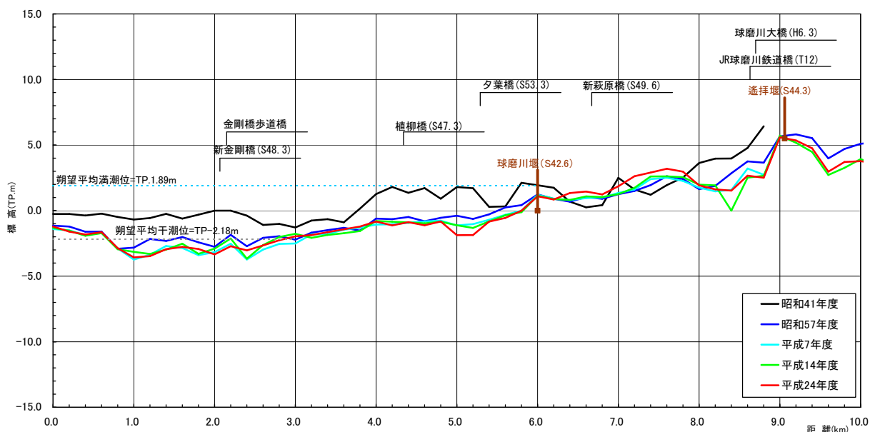
図16 球磨川下流の平均河床高縦断図
