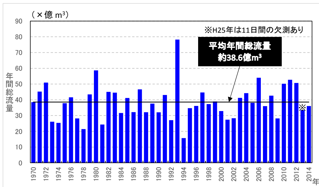
図 15 球磨川（横石）の年間総流量の推移
