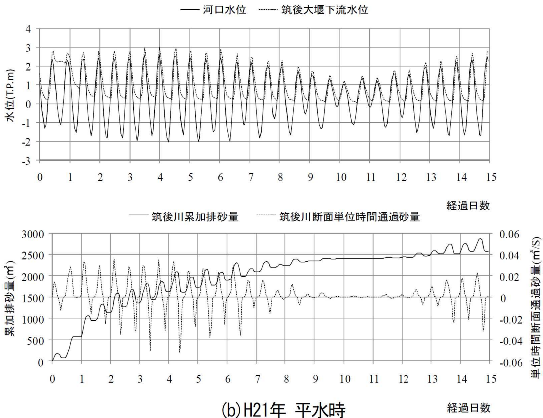
図 23 筑後川流域河床変動解析による流量時系列と有明海に流入する土砂量の推計結果
