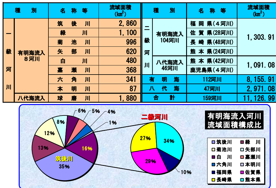
図1 有明海、八代海の流入河川の流域面積等
