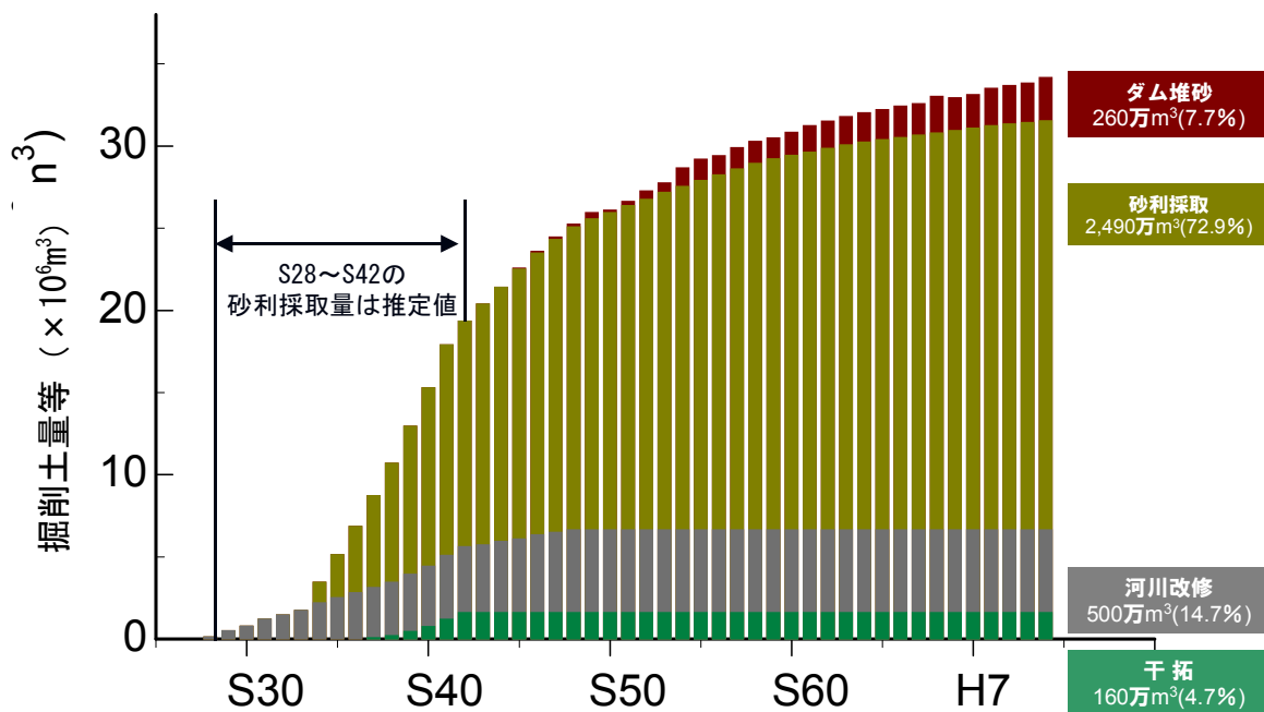
図3 河川 (筑後川) からの土砂の持出し等の累積値
