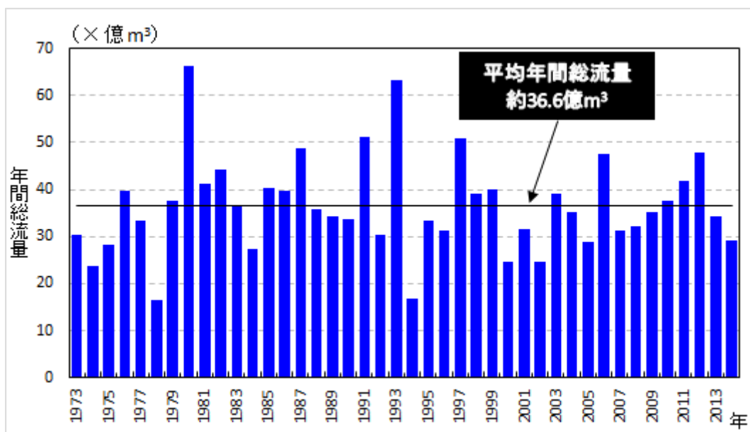
図2 筑後川（瀬の下）の年間総流量の推移
