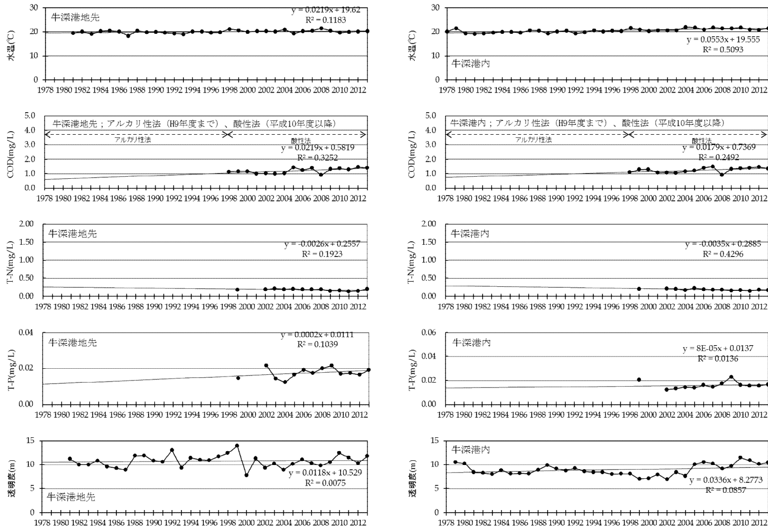
図 5 水質の経年変化[牛深港]
