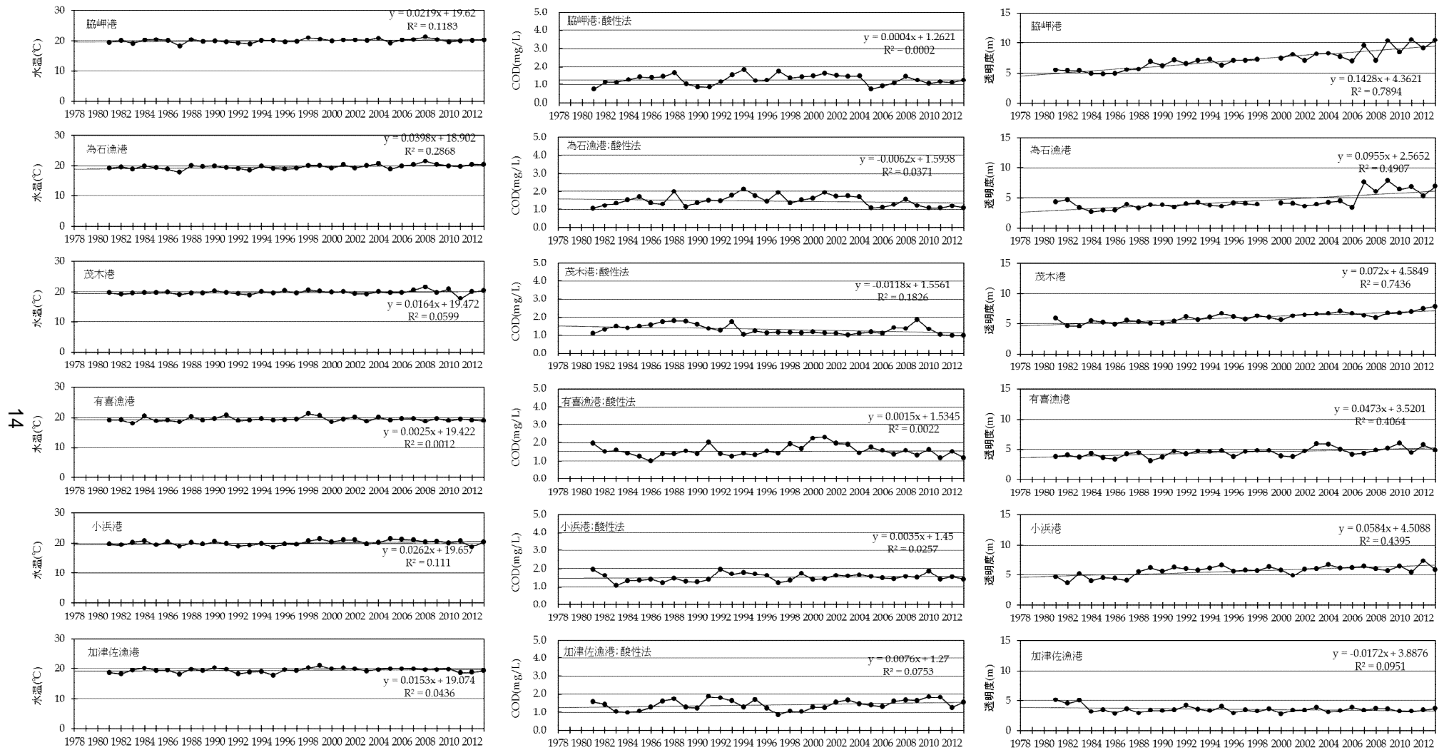
図 4 水質の経年变化[橋湾]: 水温、COD、透明度(年平均値)
