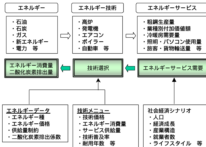
図 2 - 1 . AIM/Enduse の概要
