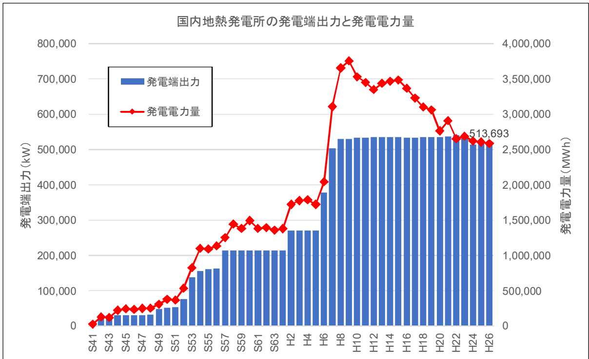
図4 国内地熱発電所の発電端と発電電力量の推移
