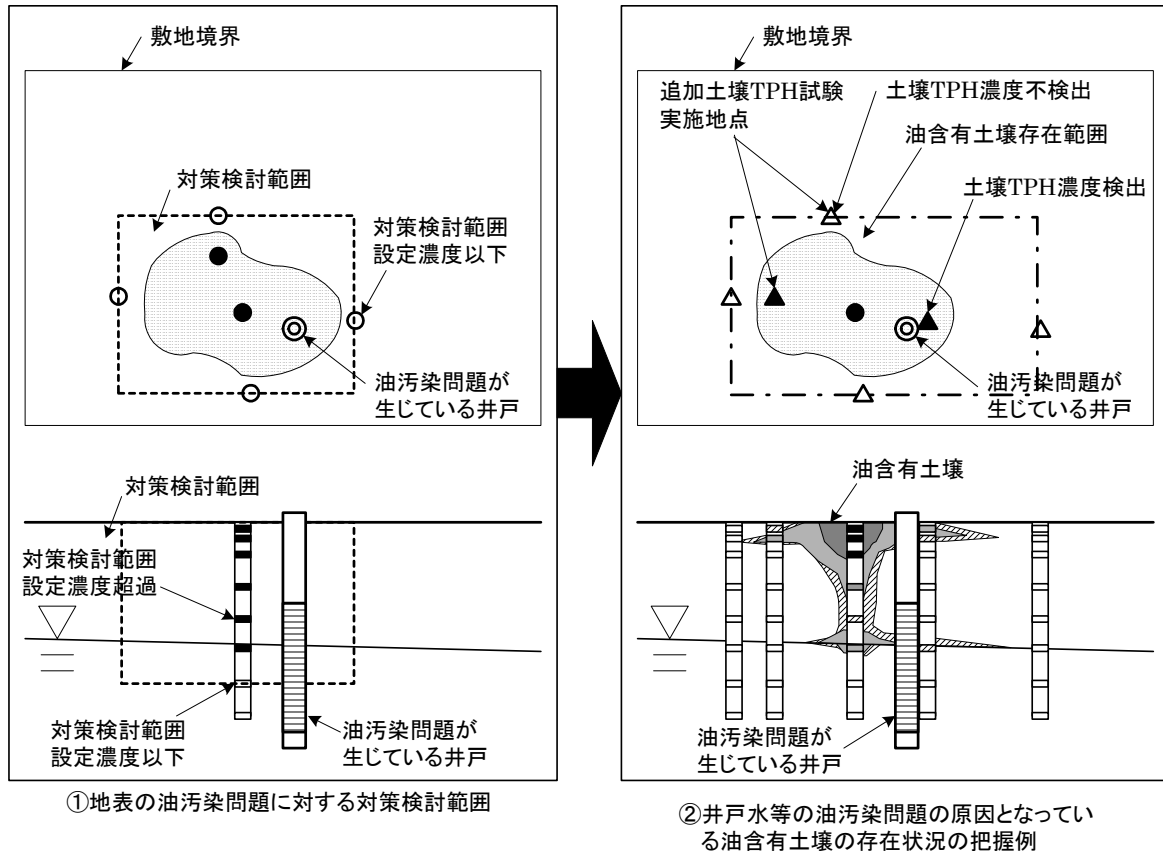
図5-2 地表と井戸水等の両方で油汚染問題が生じている場合の油含有土壤の存在状況把握の概念図
