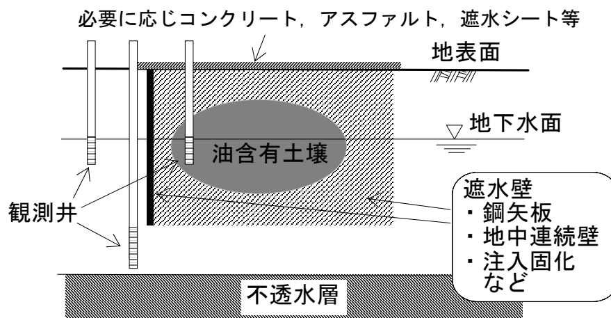
図5 遮水壁の概念図
