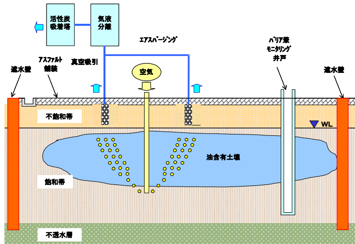
図7 エアスパージングの概念図
