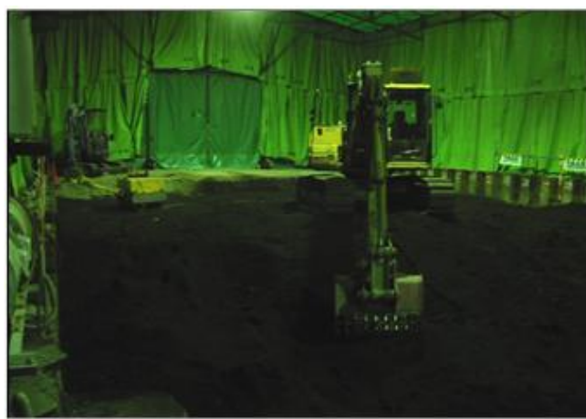
写真2 掘削除去の施工状況
