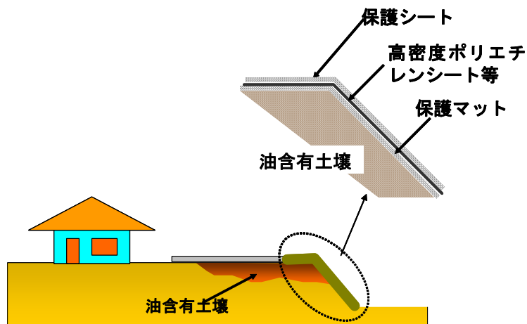
図3 シートによる被覆の概念図
