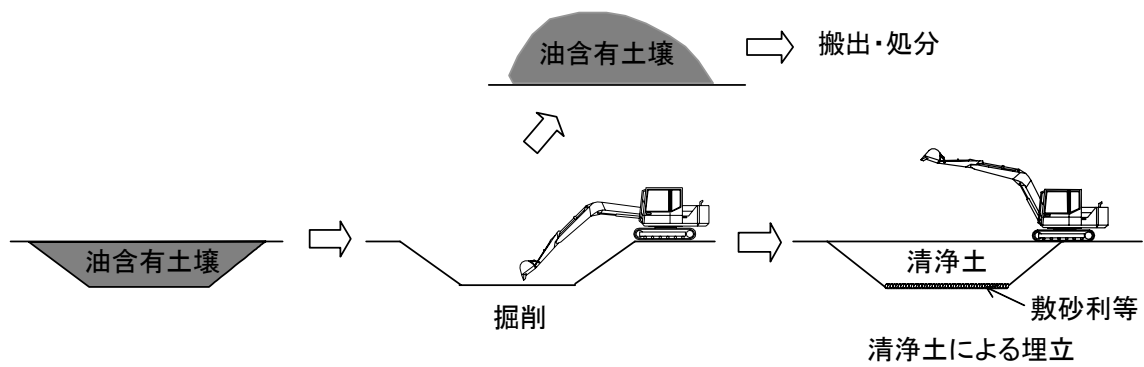
図4 掘削除去の概念図
