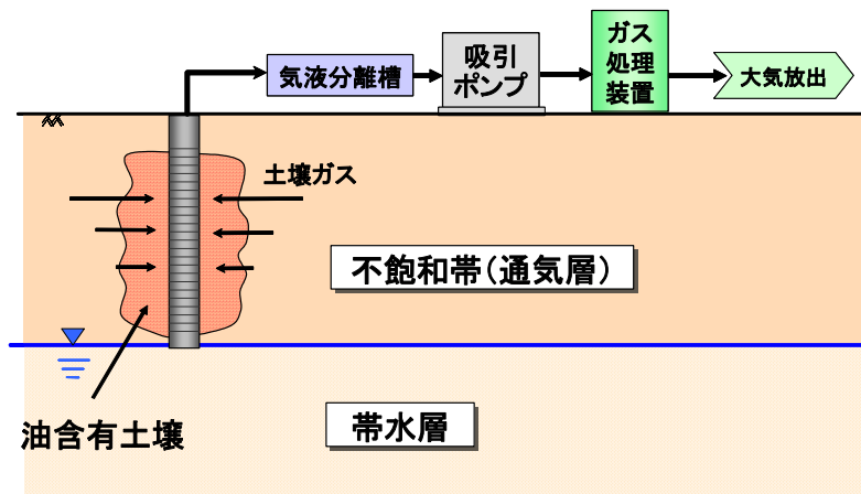
図6 土壌ガス吸引法の概念図
