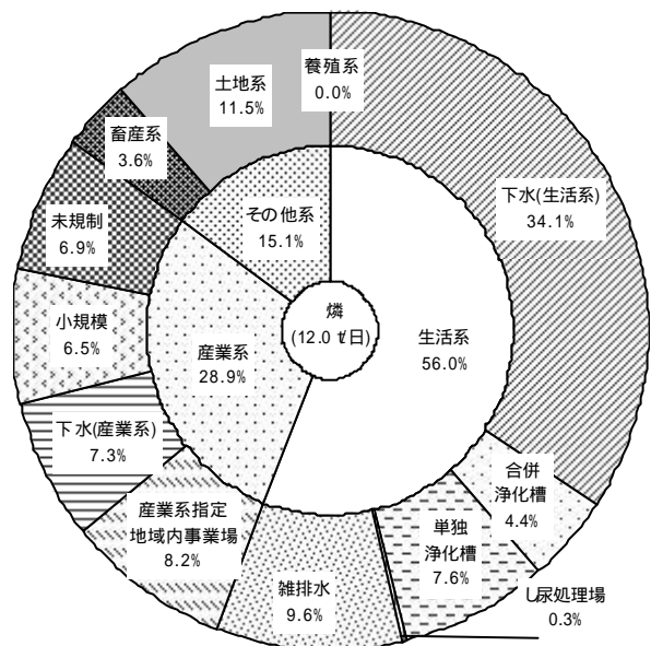
(3) 燐負荷量
