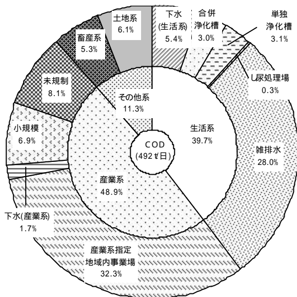
(1) COD負荷量
