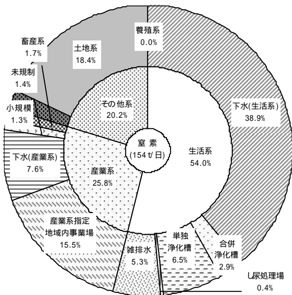
(2) 窒素負荷量
