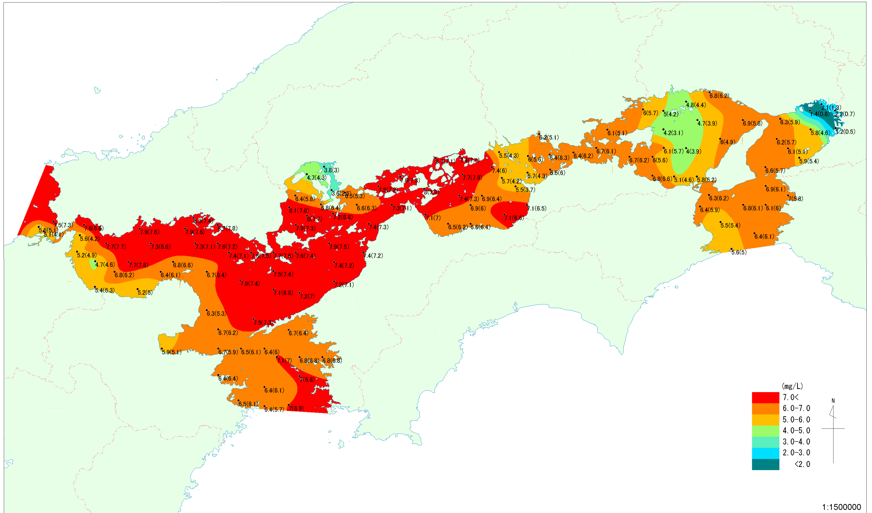
瀬戸内海におけるDOの分布 (2000~2002度 下層・夏季3ヵ年平均)
