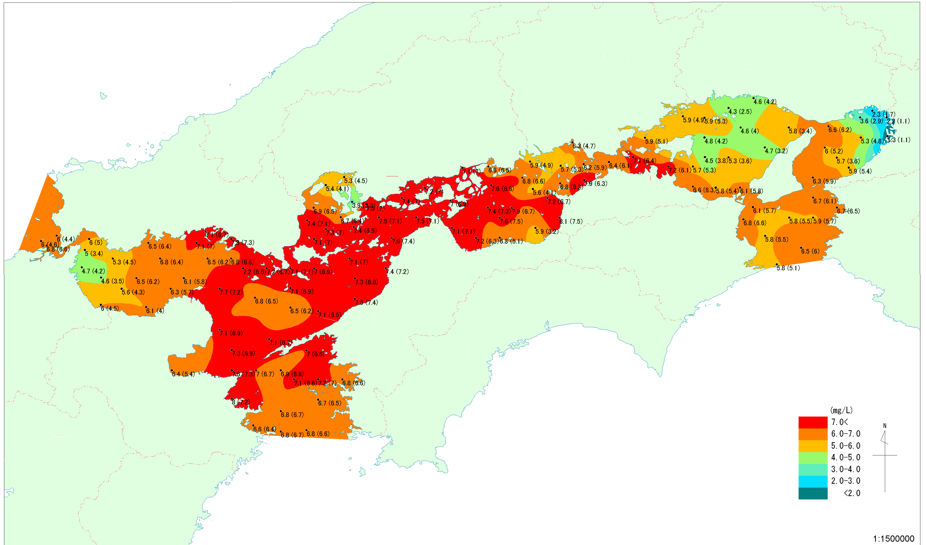
瀬戸内海におけるDOの分布 (1982~1984度 下層・夏季3ヵ年平均)
