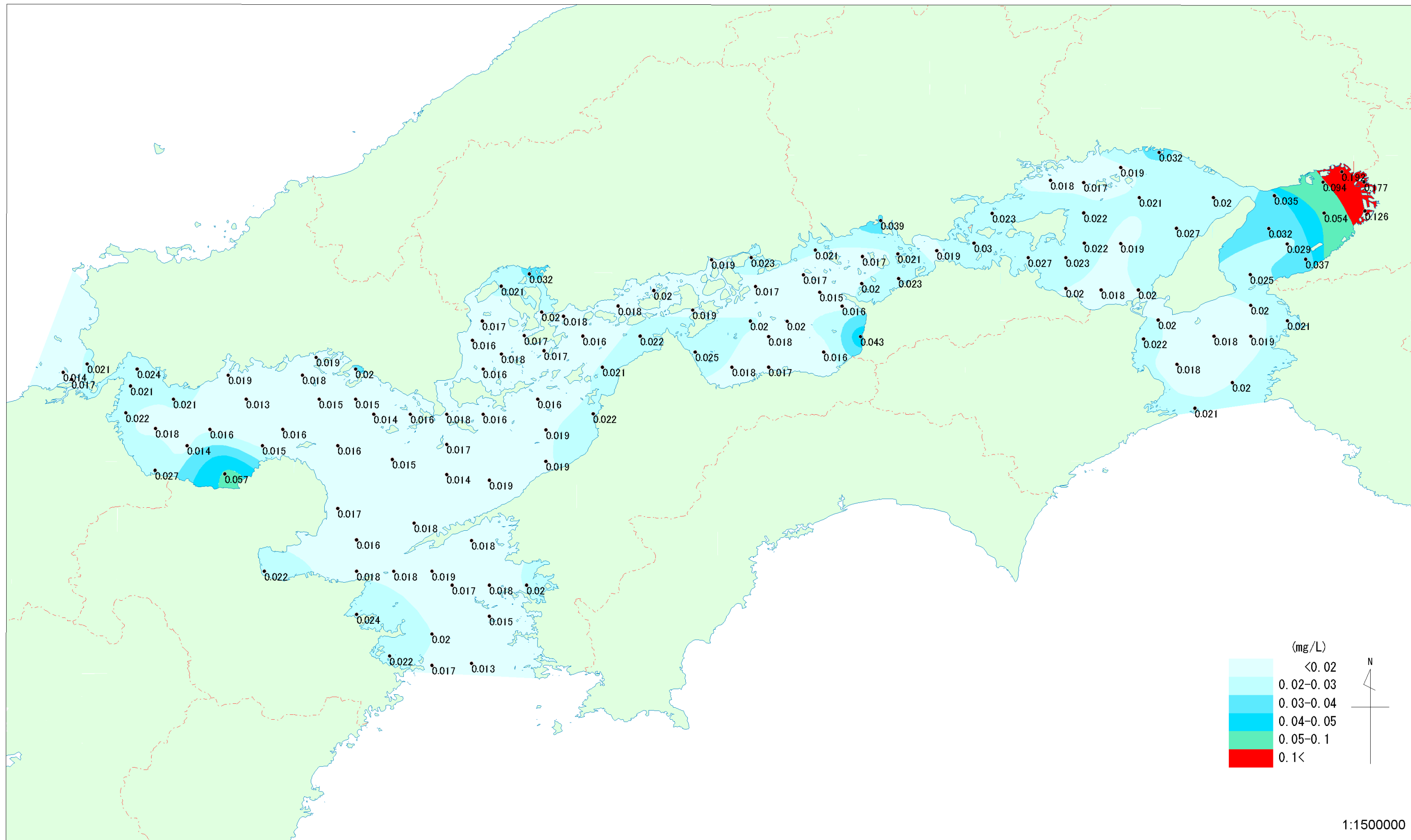
瀬戸内海におけるT-Pの分布 (1982~1984年度 上層・3ヵ年平均)
