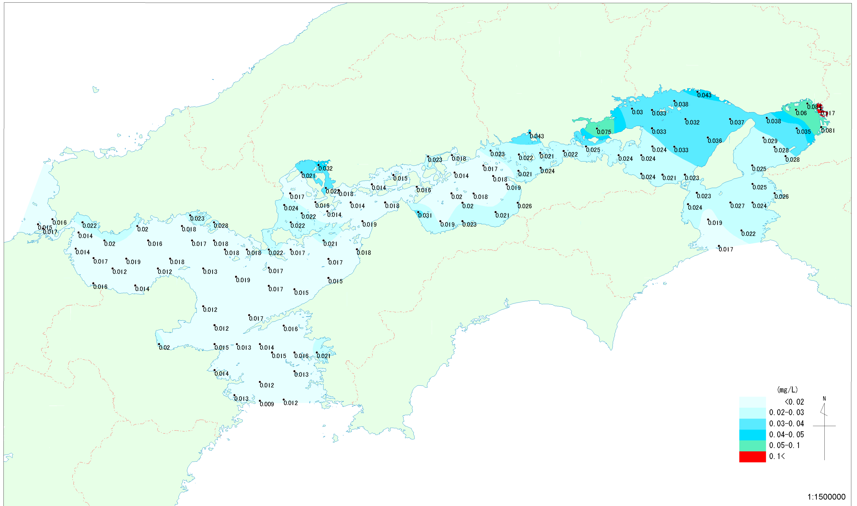
瀬戸内海におけるT-Pの分布 (2000~2002年度 上層・3ヵ年平均)
