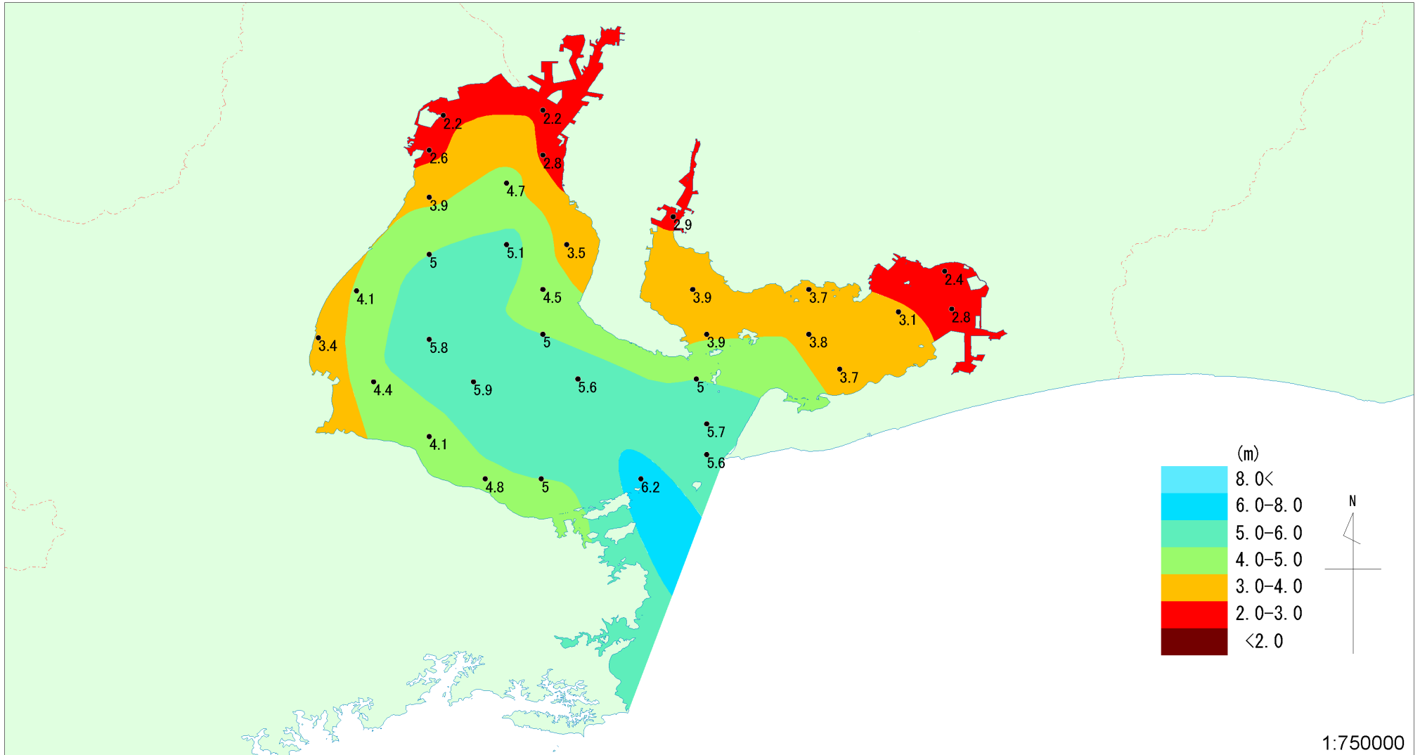
伊勢湾における透明度の分布 (1982~1984年度 上層・3ヵ年平均)
