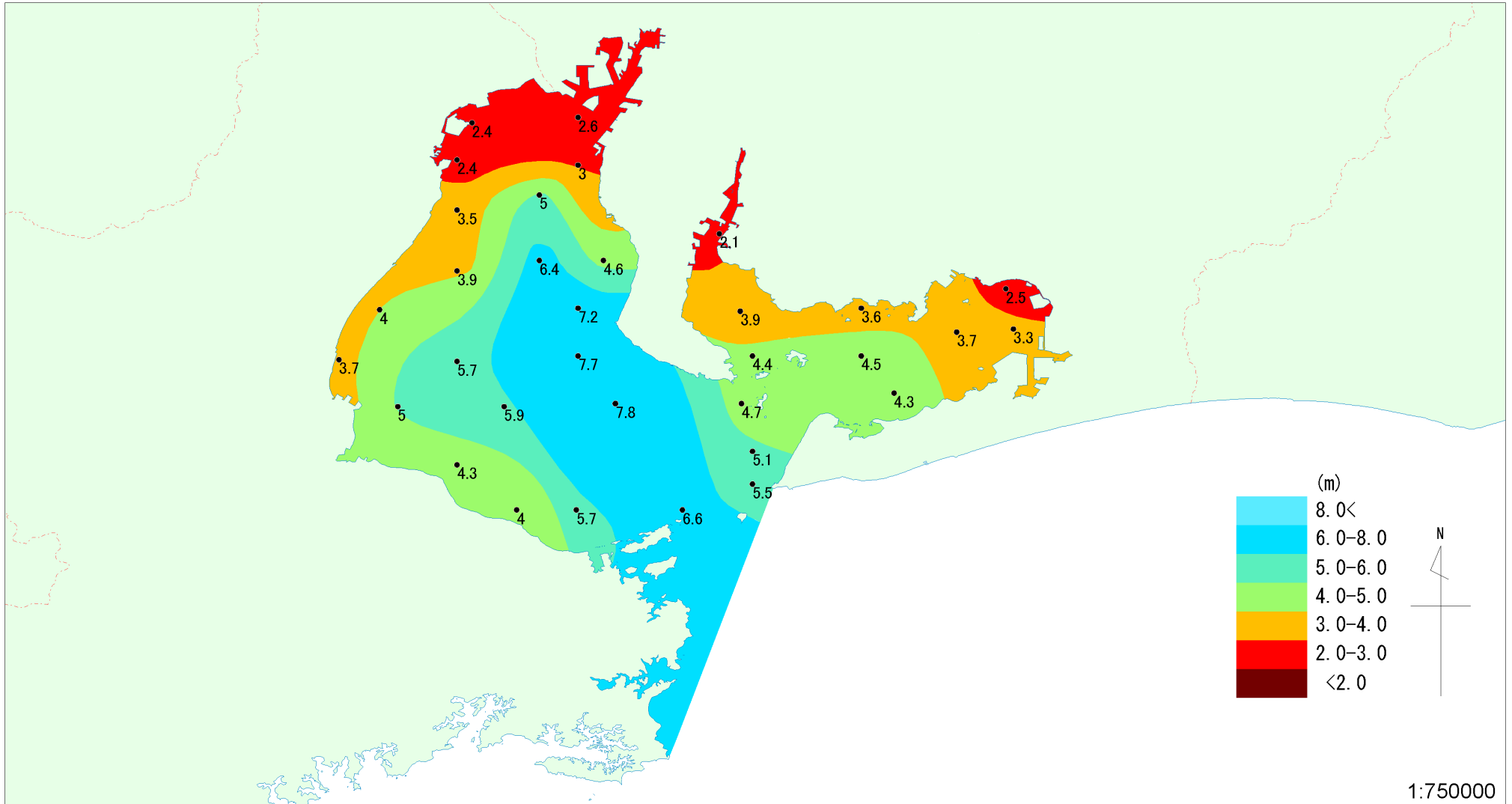
伊勢湾における透明度の分布 (2000~2002年度 上層・3ヵ年平均)
