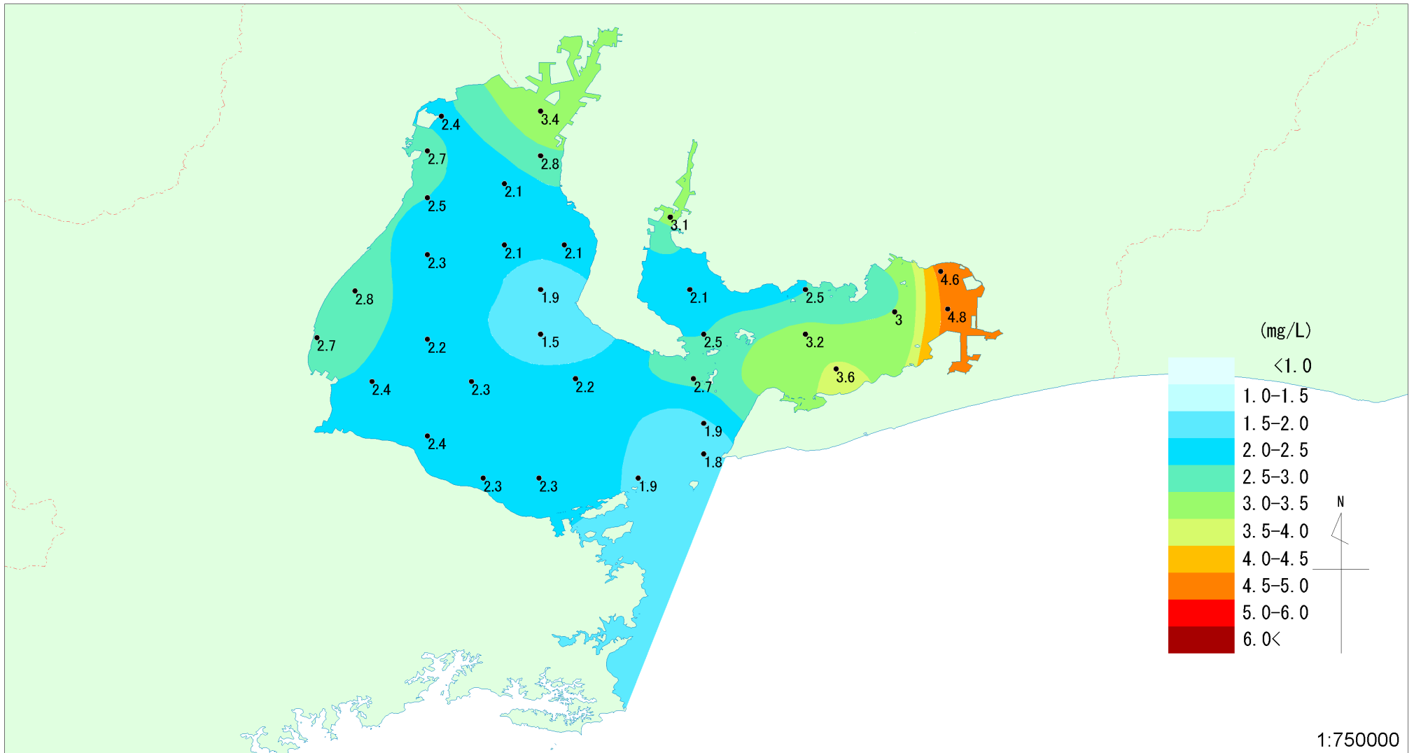
伊勢湾におけるCODの分布 (1982~1984年度 上層・3ヵ年平均)
