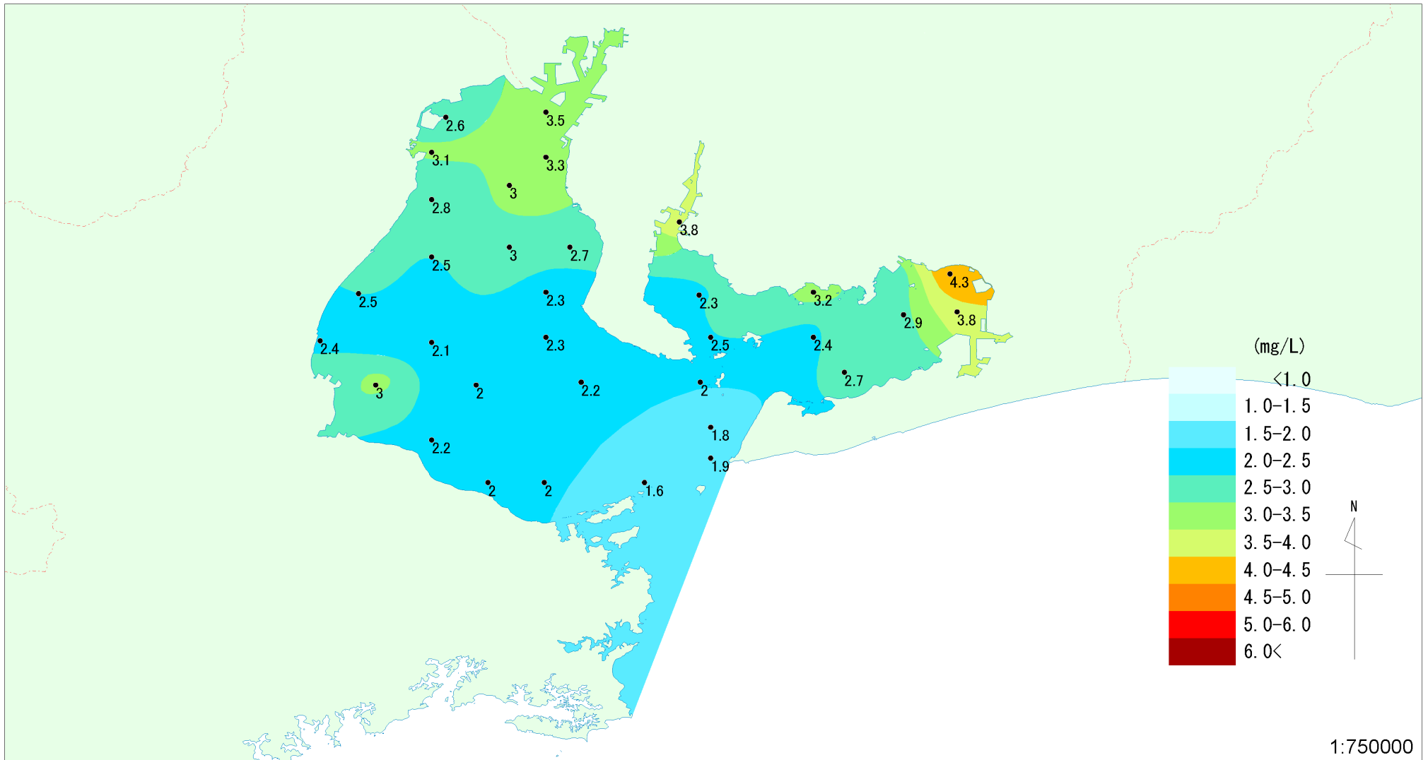
伊勢湾におけるCODの分布 (2000~2002年度 上層・3ヵ年平均)
