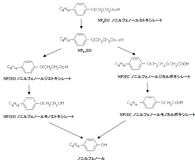
図 2 ノニルフェノールエトキシレートの分解過程( 1 )
