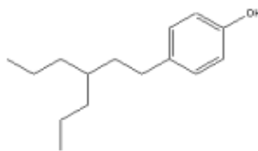
図 1 4 (又は p) - ノニルフェノール (分岐型) の構造式の一例
