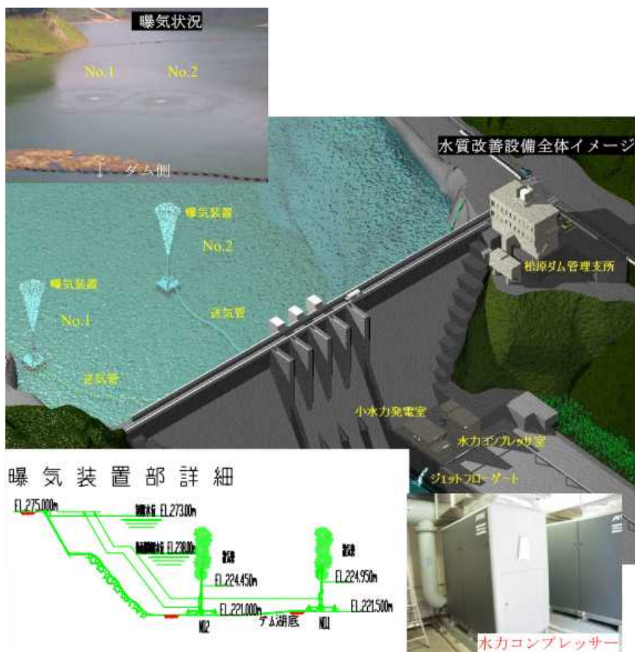
図 6.3.6 松原ダム貯水池水質改善設備（ばっ気装置）
