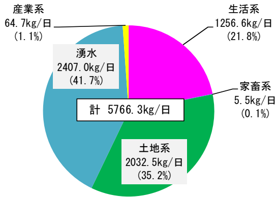
相模ダム(T-N)：現況・平成22年度
