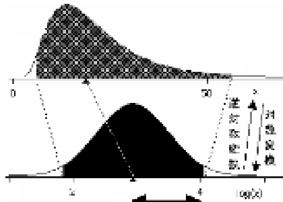
正規分布と対数正規分布の標準的な分布波形
