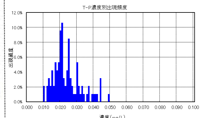
荒川貯水池の水質測定データの濃度分布 (平成10年度～平成17年度)
