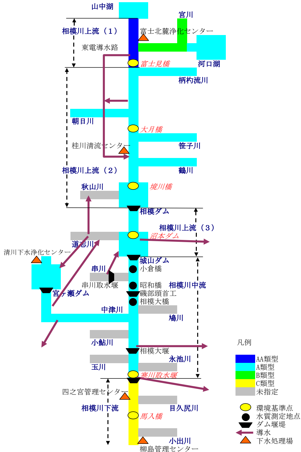
図 8.17 相模川水系導水概要図
