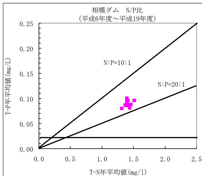
図 8.4 相模ダム N/P 比の状況
