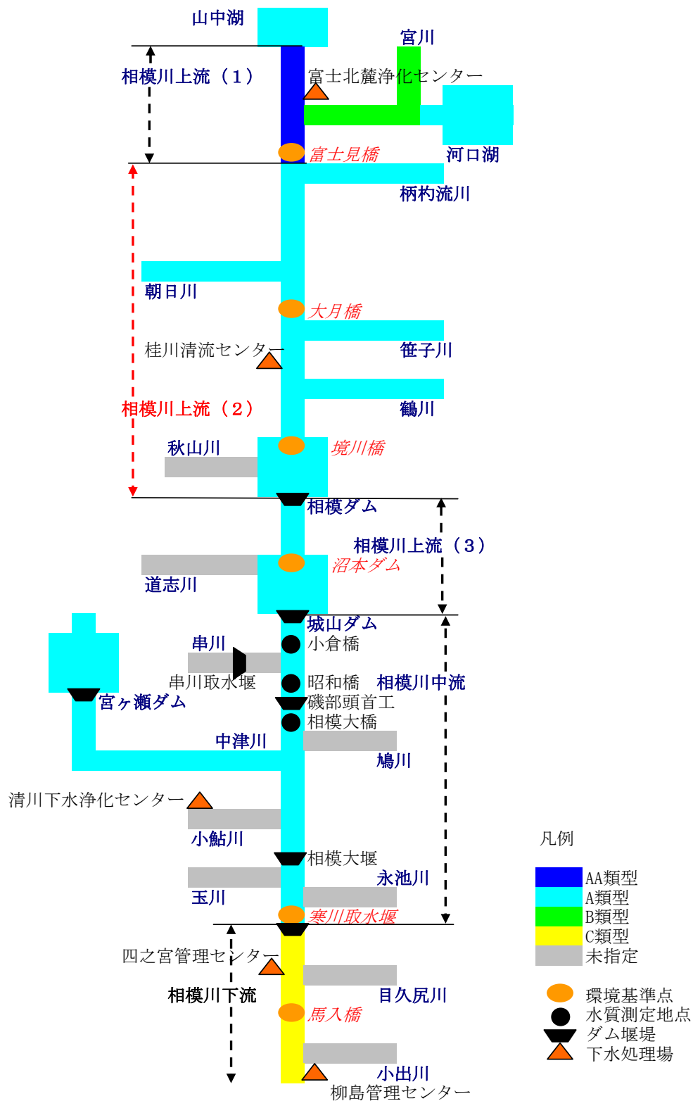
図 8.2 相模ダム流域の概要図
