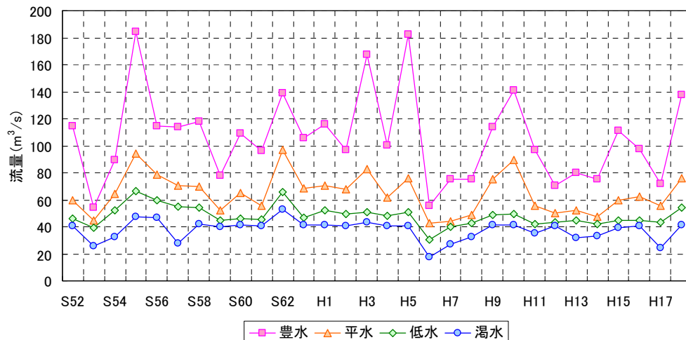
図 3.5 瀬ノ下の流量経年変化
