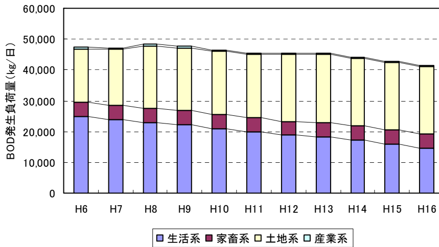
図 3.17 筑後川(3) BOD 発生負荷量の推移
