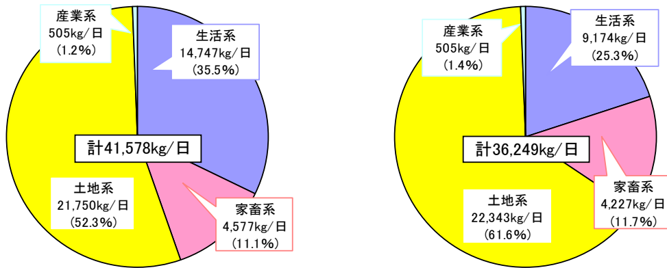
図 3.16 筑後川(3)のBOD 発生汚濁負荷量
