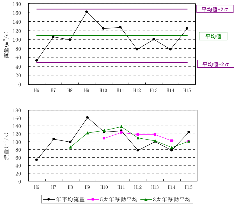
図 3.18 筑後川（3）の流量の経年変化
