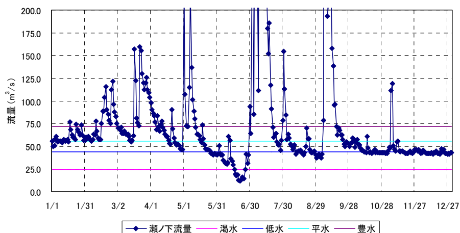
図 3.6 瀬ノ下流況（平成 17 年）
