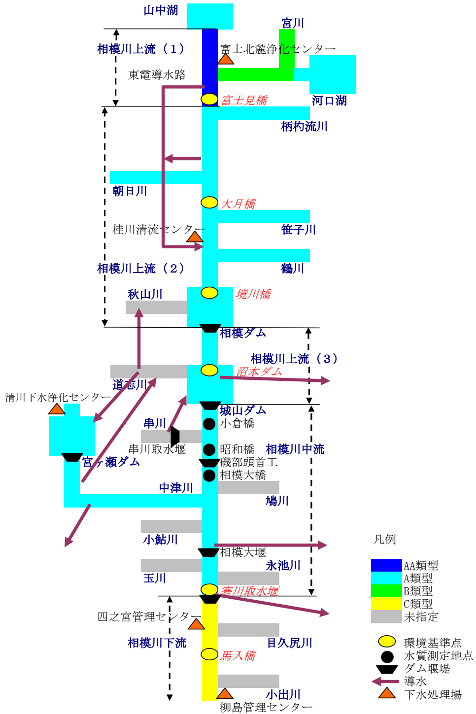
図 2.21 相模川水系導水概要図
