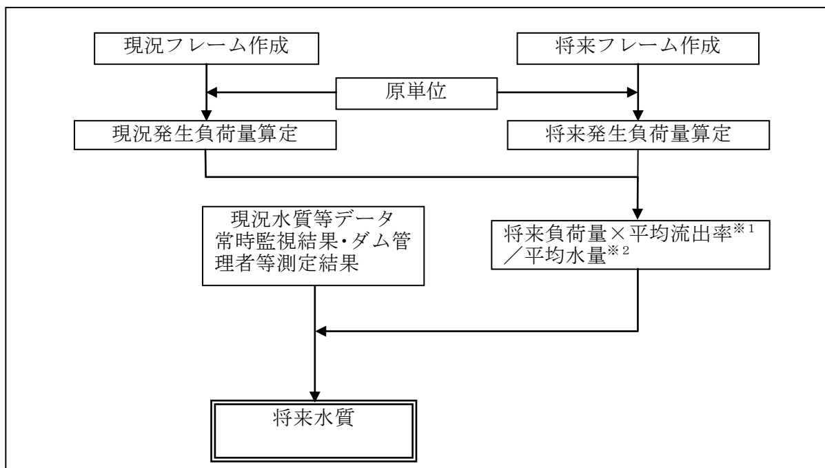
図 2.20 城山ダム貯水池の水質予測手法
