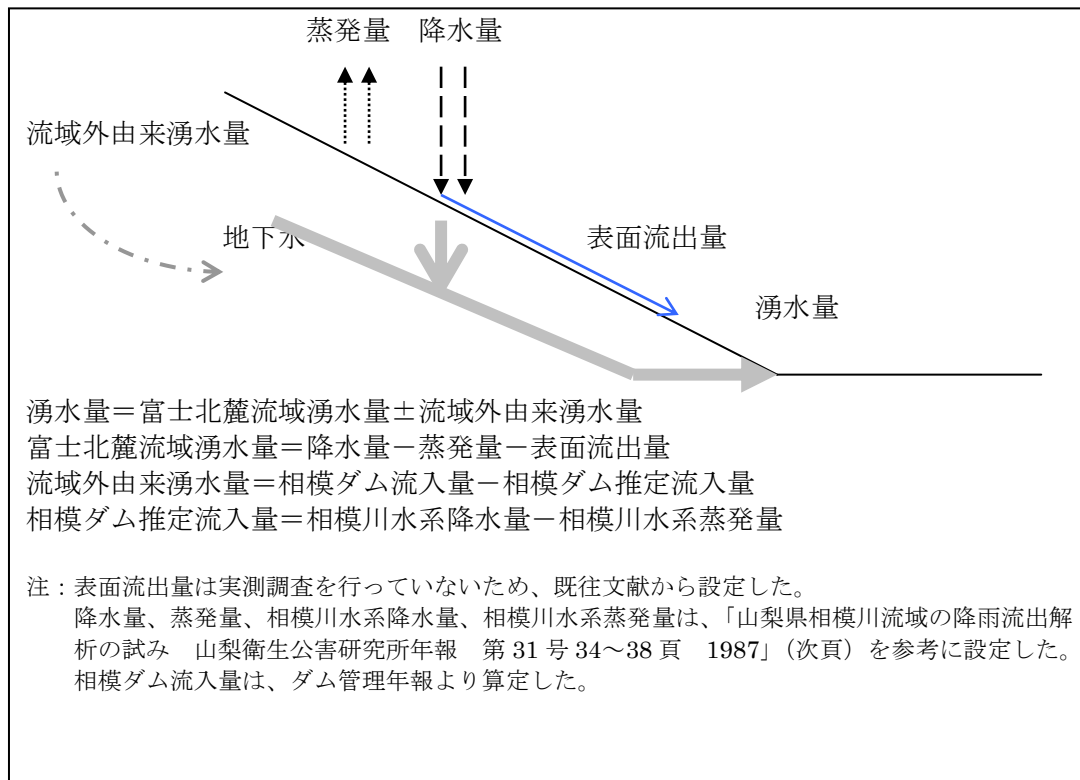
図 2.17 湧水負荷量の算定方法
