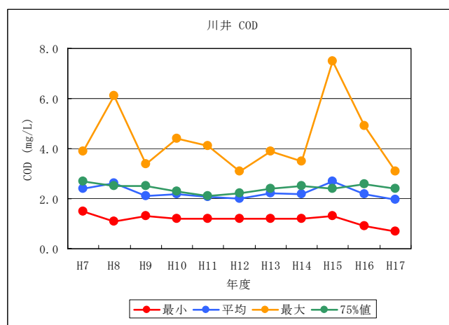
図 2.17 土師ダム貯水池流入水質 (COD) の推移
