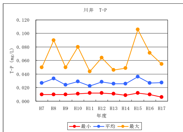
図 2.20 土師ダム貯水池流入水質 (T-P) の推移
