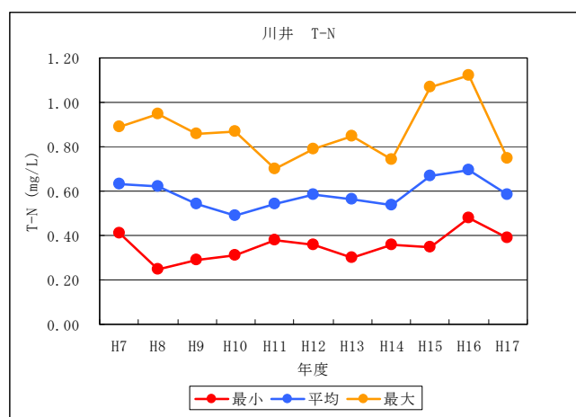
図 2.19 土師ダム貯水池流入水質 (T-N) の推移
