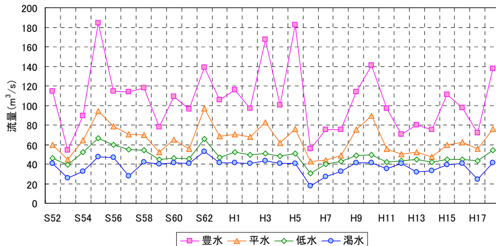
図 2.5 瀬ノ下の流量経年変化
