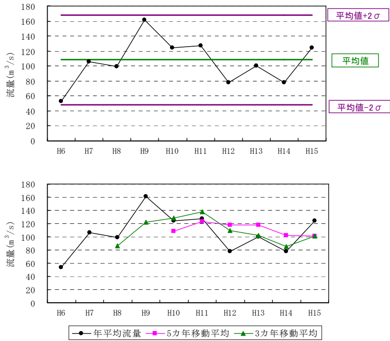
図 2.16 筑後川 (3) の流量の経年変化
