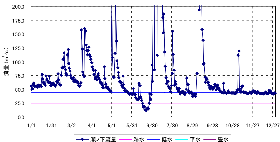
図 2.6 瀬ノ下流況（平成17年）
