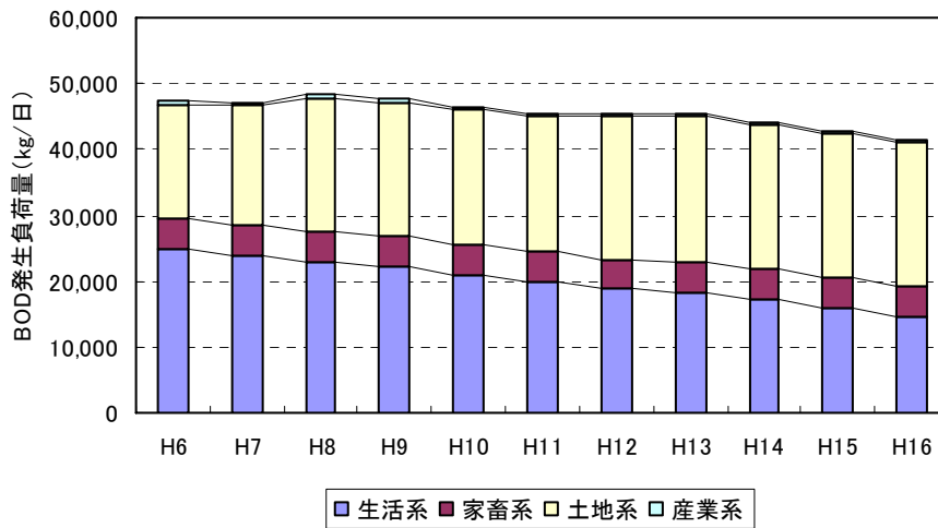
図 2.15 筑後川(3) BOD発生負荷量の推移
