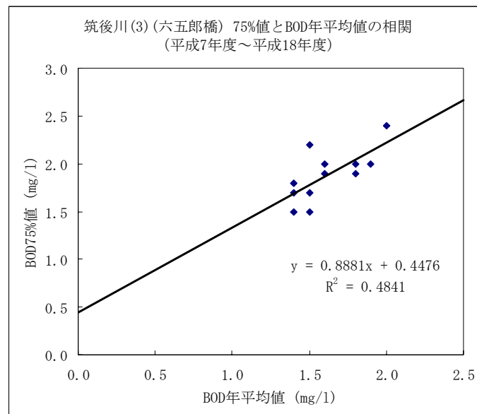
図 2.17 筑後川(3)水域（六五郎橋）の BOD 年平均値と 75%値
