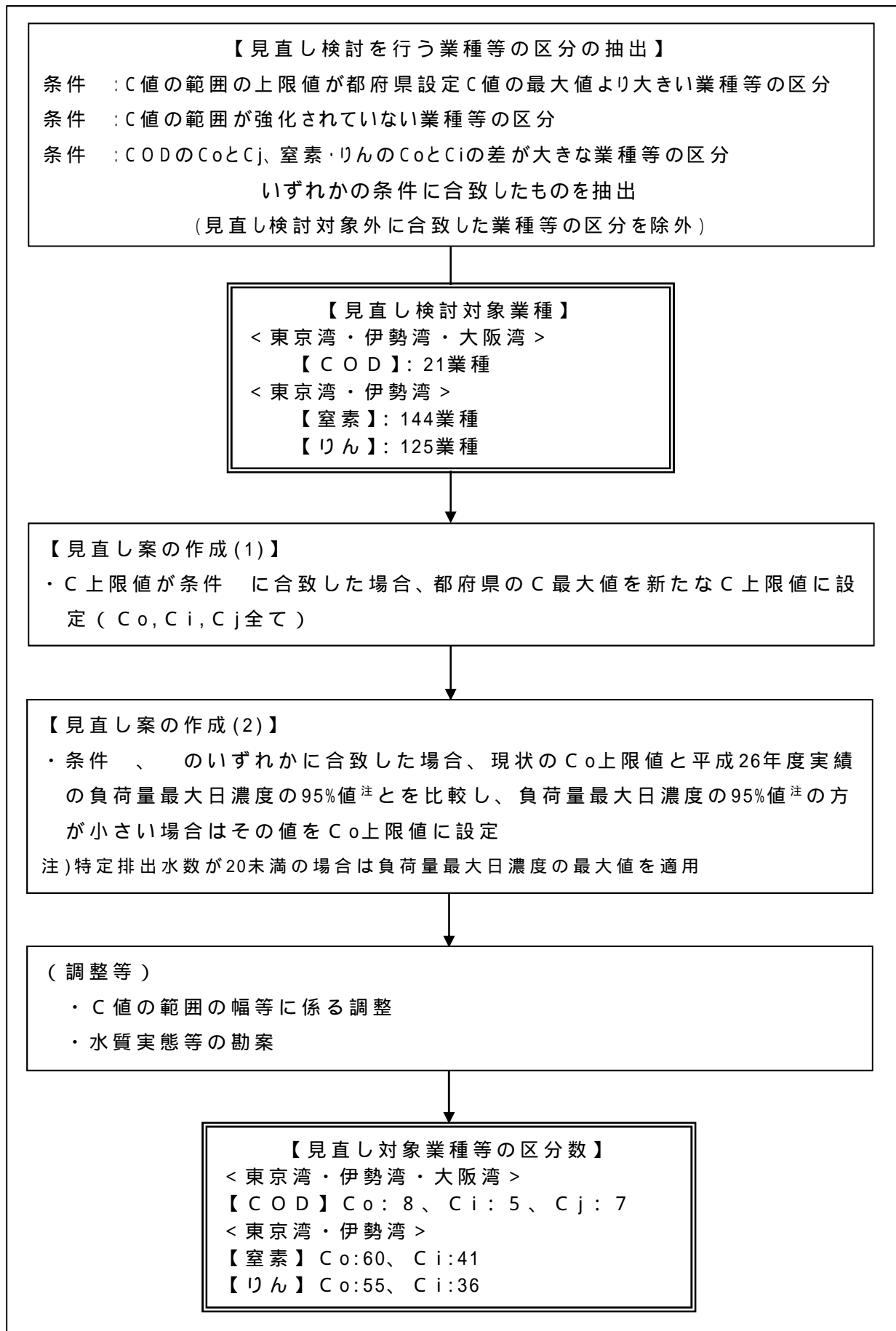
図 C 値の範囲の見直し案作成手順 (概要) と見直し対象業種等の区分数
