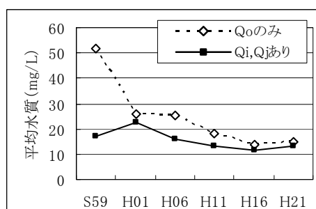
図1. 「Q o のみのもの」の水質が「Q i 、Q j を含むもの」と同様の値を示す場合
