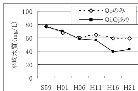
図2. 「Q o のみのもの」の水質の改善の度合いが少ない場合
