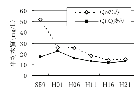
図1. 「Q o のみのもの」の水質が「Q i、Q j を含むもの」と同様の推移を示す場合
