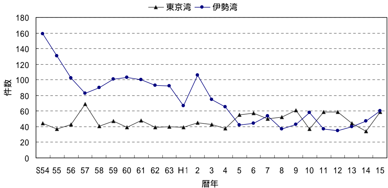
図 1 8 東京湾及び伊勢湾における赤潮の発生状況
