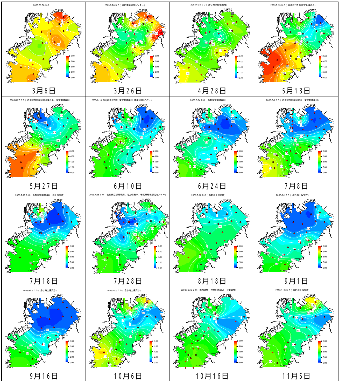
図 2 1 東京湾における底層DO(m / )の分布 (平成 15 年)
