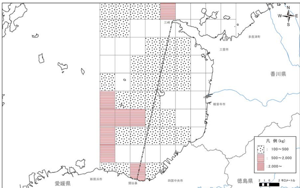
出典：水産庁：漁場環境評価メッシュ図，瀬戸内海（平成 11 年 3 月）より作成 図 3.10(6) 主要魚種の漁場分布図（クルマエビ）
