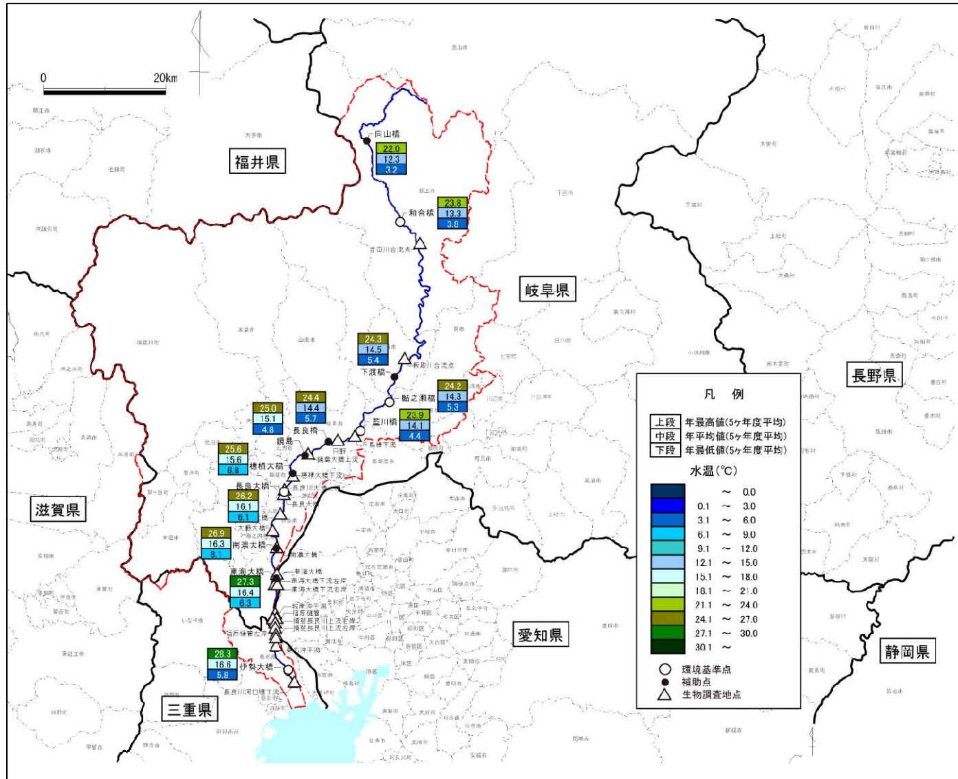
図 2.78 水温(長良川)
