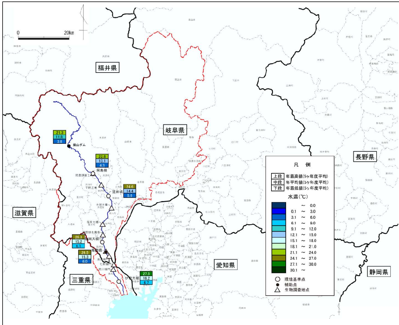
図 5.8 水温(揖斐川)
