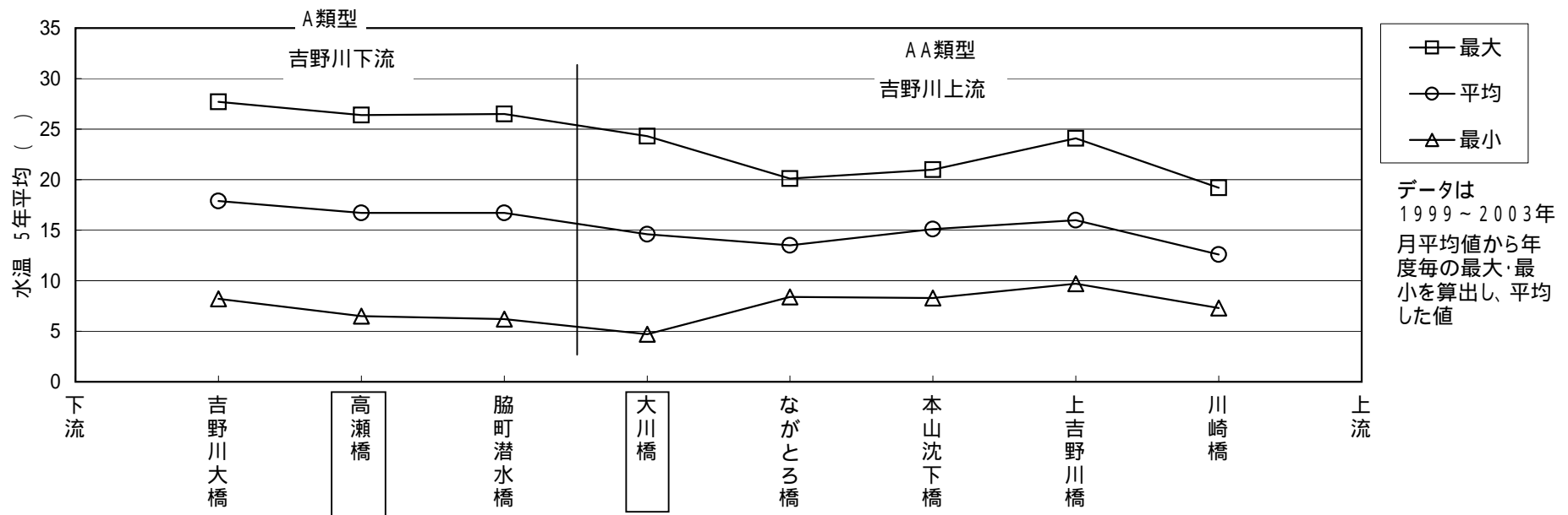
図3.4.8 水温の水質縦断分布
