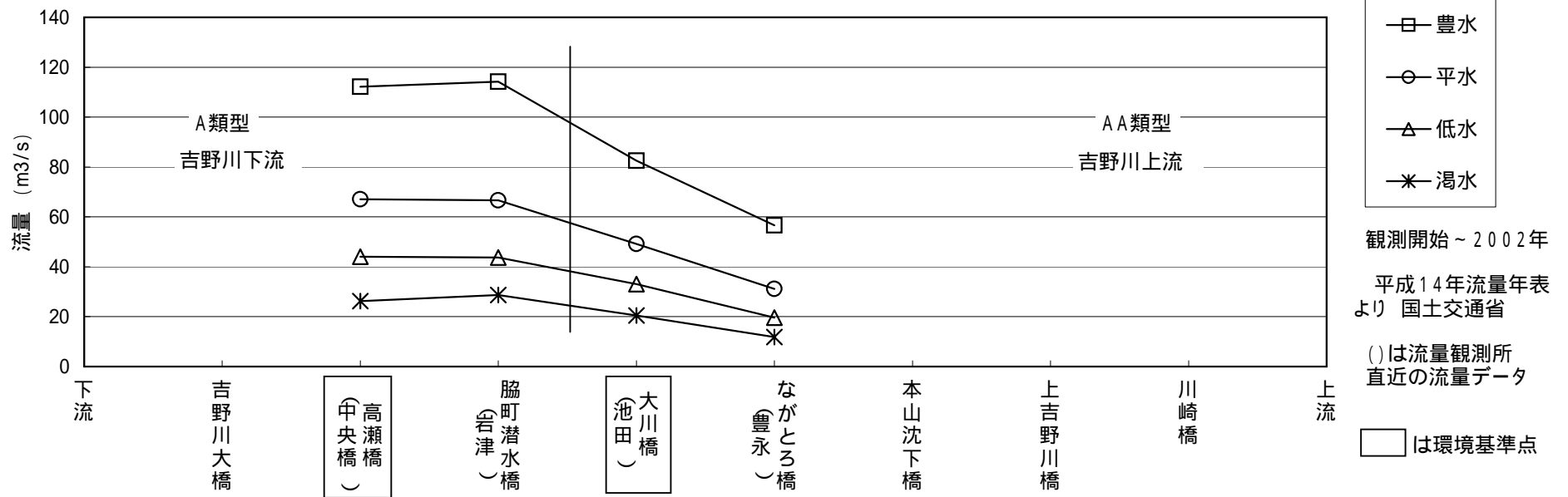
図3.4.10 流量の縦断分布
