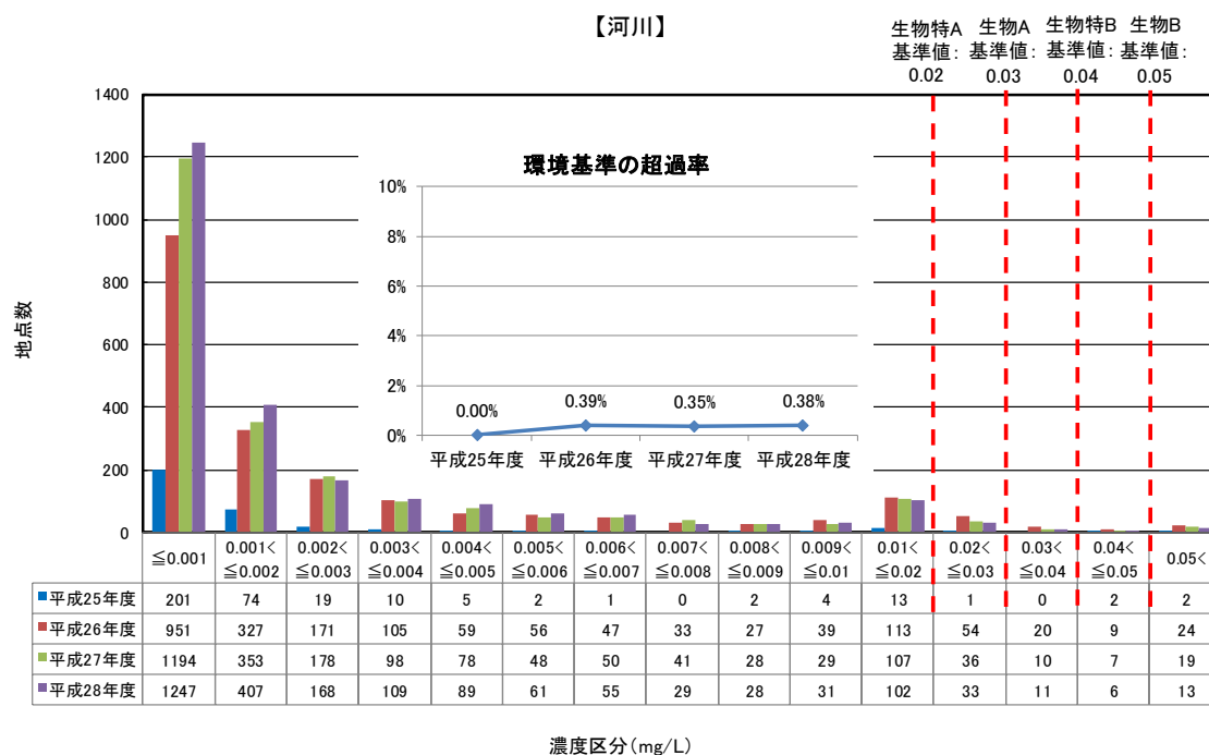
図 1 公共用水域(河川)におけるLASの調査地点数及び検出濃度の分布 1)
