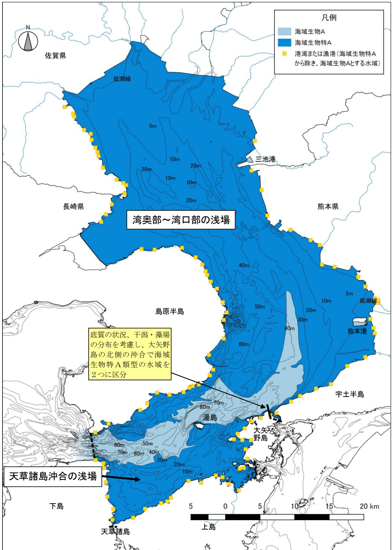
図1 有明海における海域生物A、海域生物特Aの類型指定（案）
