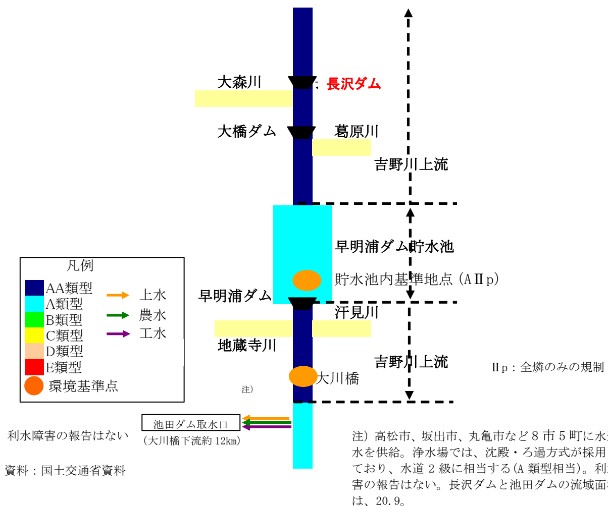
図 3.4.1 長沢ダム流域の利水状況
