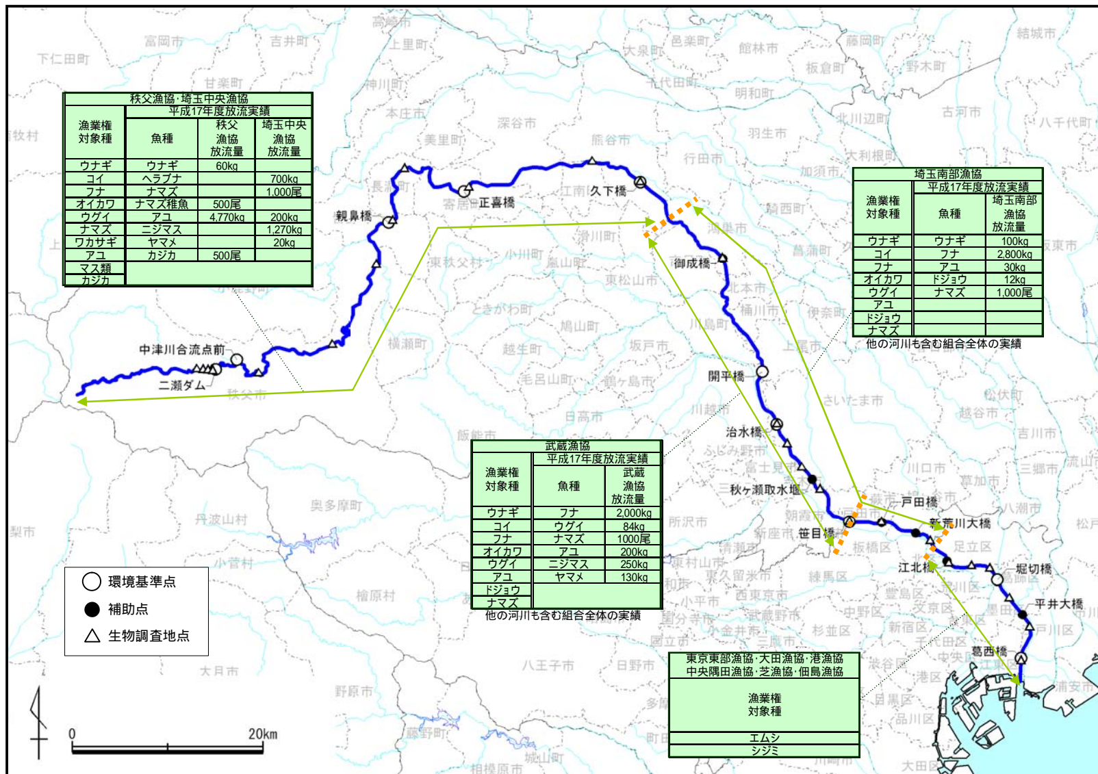
図8.12 荒川【漁業権設定・魚類等放流状況】
